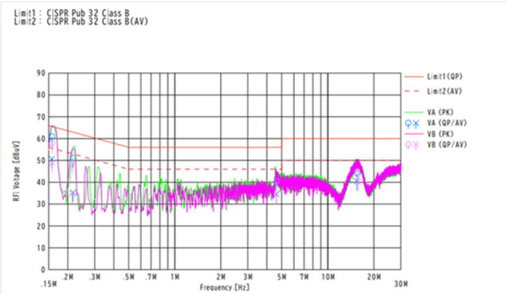
Figure 23. V_{IN} : 115 Vac / 60 Hz, I_{OUT} : 4.5 A
