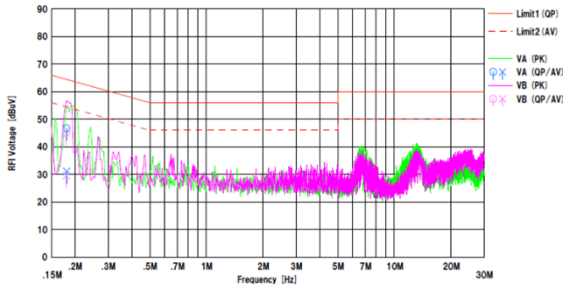
Figure 24. V_{IN} : 115 Vac / 60 Hz, I_{OUT} : 2 A
