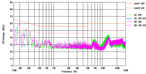
Figure 23. V_{IN} : 230 Vac / 50 Hz, I_{OUT} : 2 A
