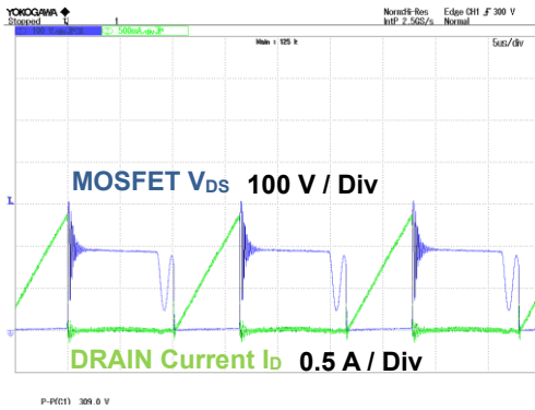
Figure 11. V_{DS} , I_D V_{IN} = 90 Vac, I_{OUT} = 2 A
