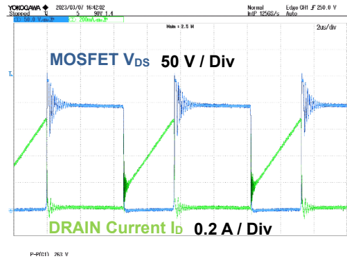
Figure 11. V_{DS} , I_D V_{IN} = 90 Vac, I_{OUT} = 1.4 A
