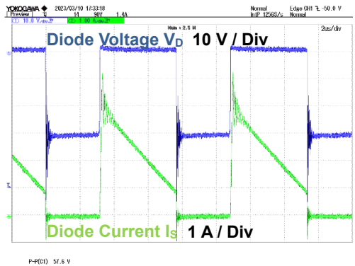
Figure 13. V_D , I_S V_{IN} = 90 Vac, I_{OUT} = 1.4 A
