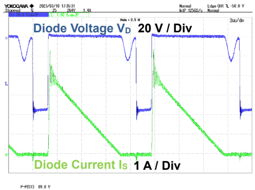
Figure 14. V_D , I_S V_{IN} = 264 Vac, I_{OUT} = 1.4 A
