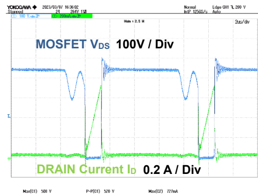
Figure 12. V_{DS} , I_D V_{IN} = 264 Vac, I_{OUT} = 1.4 A
