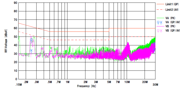
Figure 24. V_{IN} : 115 Vac / 60 Hz, I_{OUT} : 1.4 A
