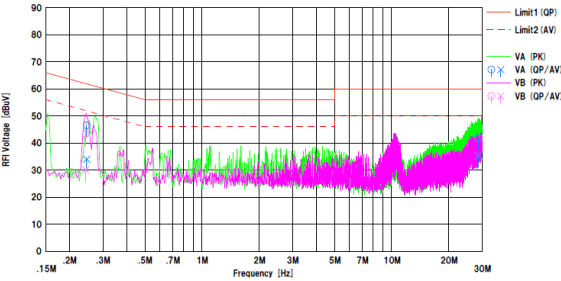
Figure 23. V_{IN} : 230 Vac / 50 Hz, I_{OUT} : 1.4 A
