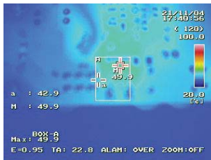
Diode 49.9 °C
