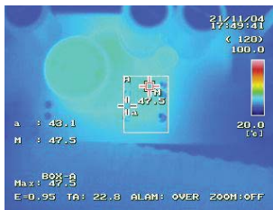
IC 47.5 °C
