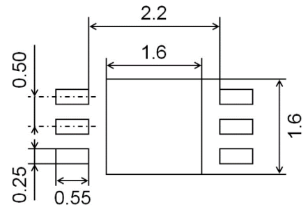
Footprint dimensions
