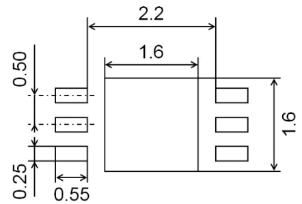
Footprint dimensions
