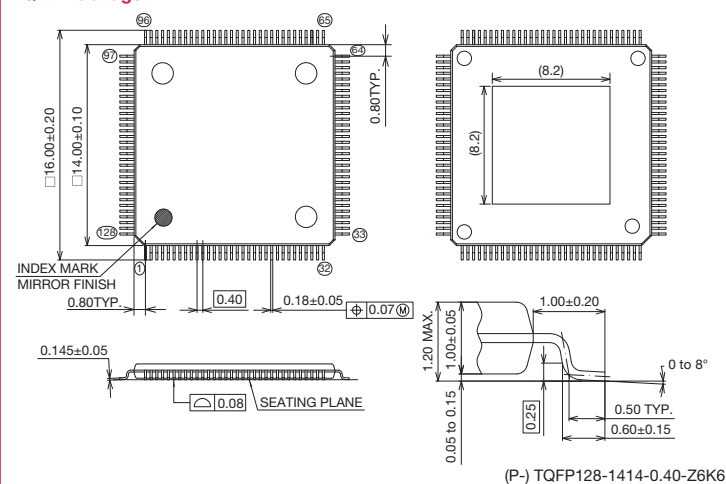
TQFP Package
