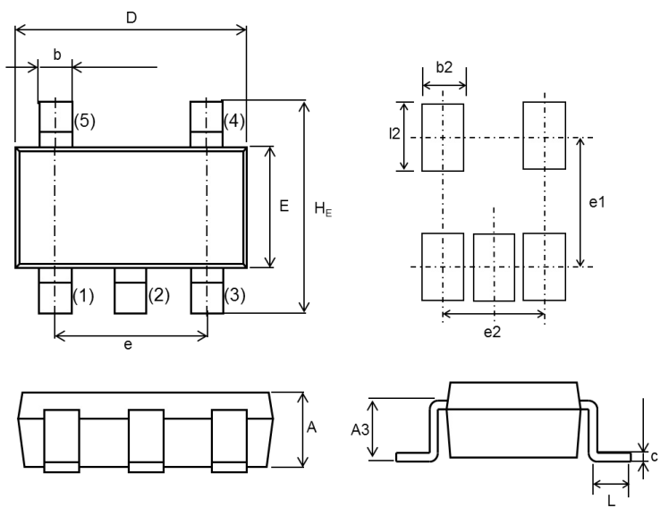
SOT-25T, (TSMD5)
