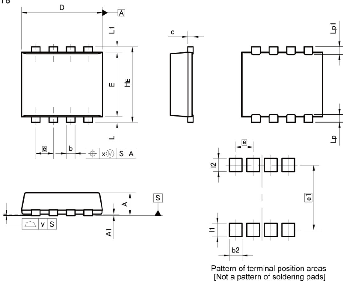
TSMT8
