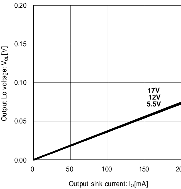
Fig. 20 Output Lo voltage ( T_a=25^\circ C )
