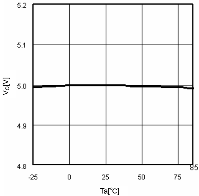
Fig.8 T_a-V_O (I_o=0mA)
