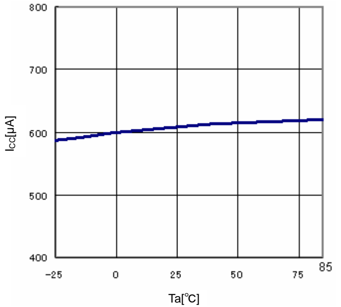
Fig.9 T_a-I_{cc}
