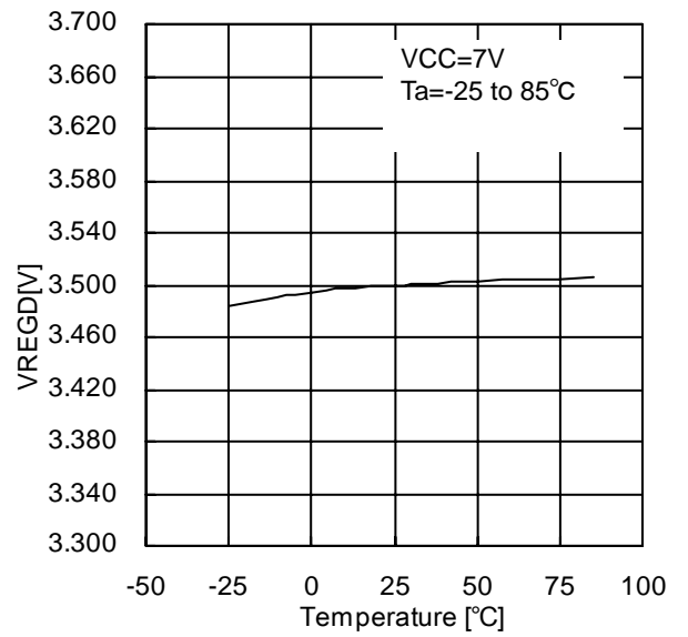
Figure.17 VREGD – Ta
