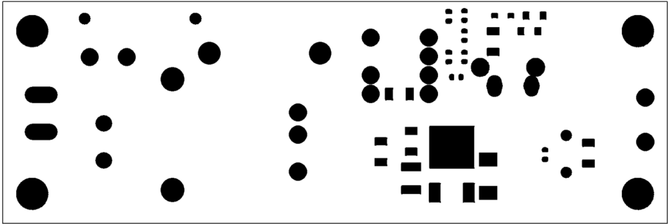
Bottom_Mask
