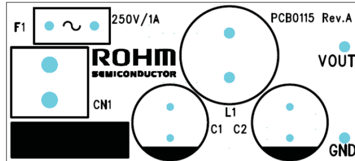
Top Layer
