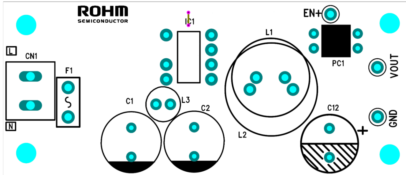
Top Layer
