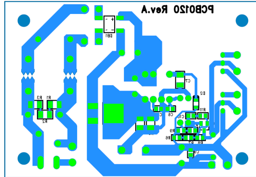
Bottom Layer
