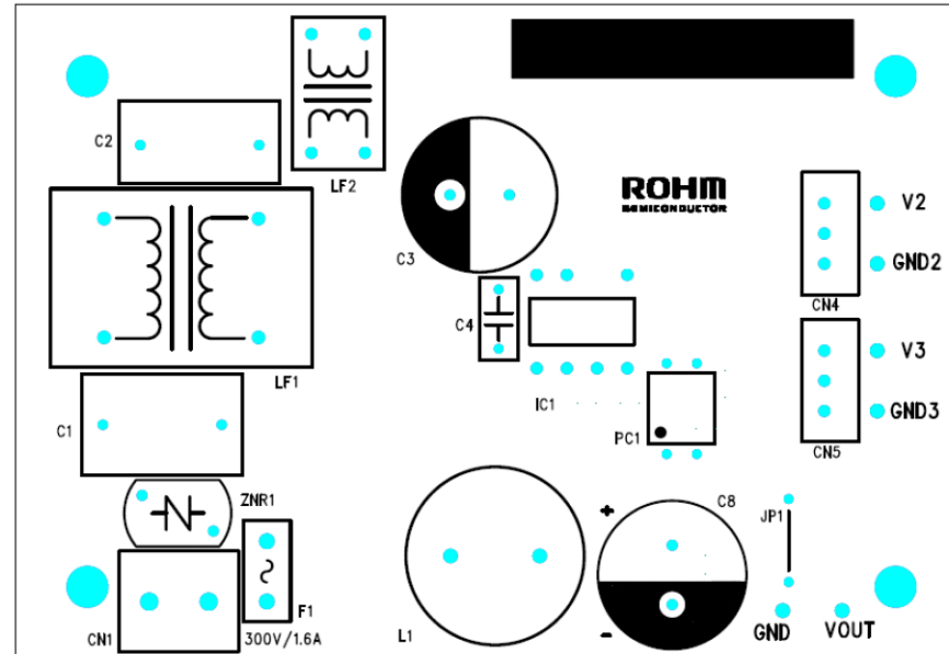
Top Layer
