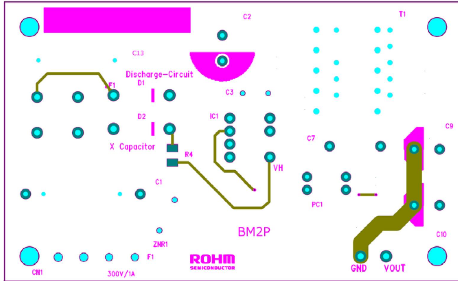
Top Layer
