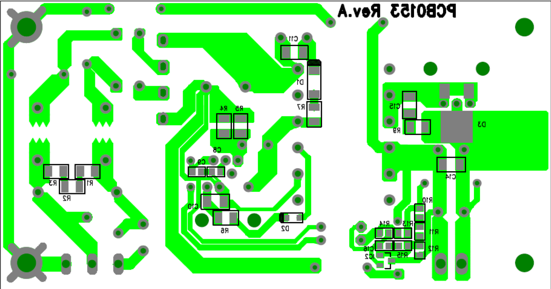
Bottom Layer
