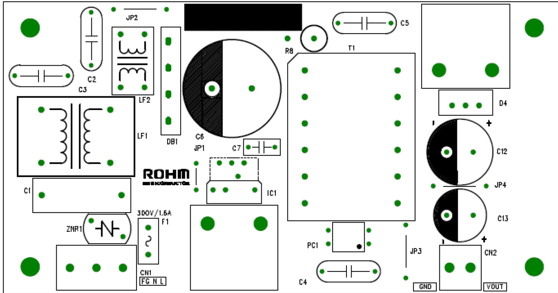
TOP Layer
