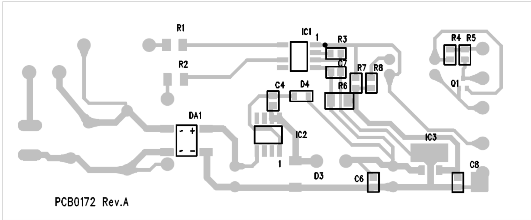
Bottom Layer
