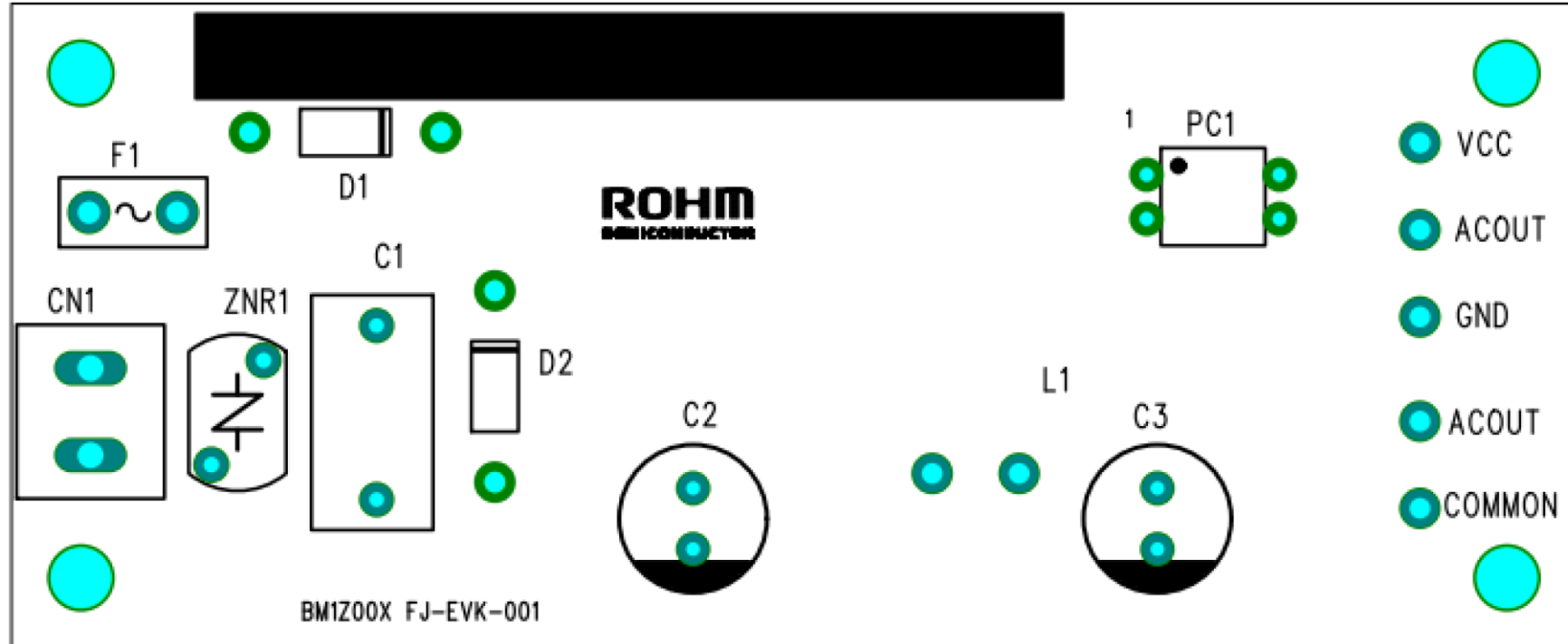
Top Layer
