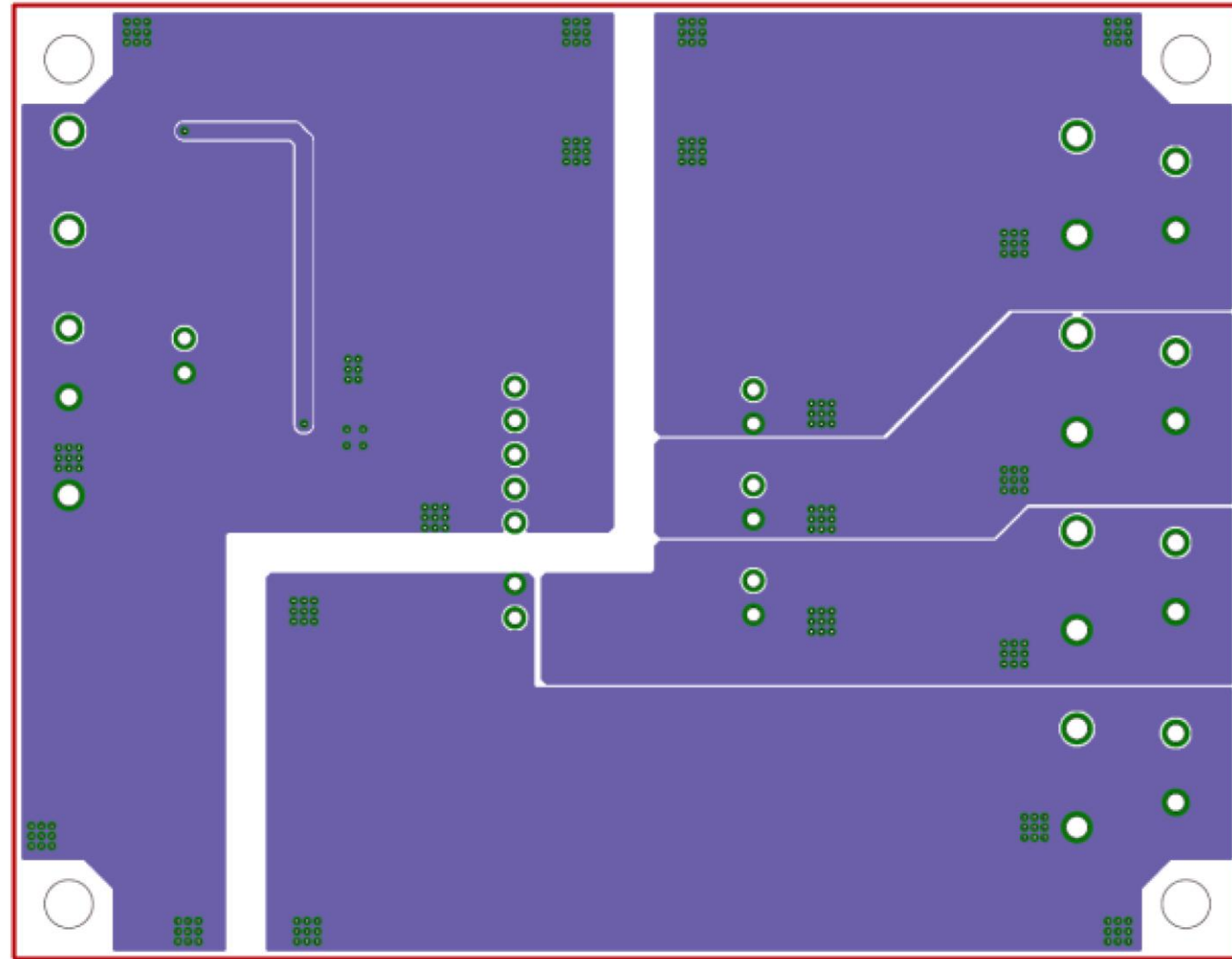
Bottom Side Layer Layout
