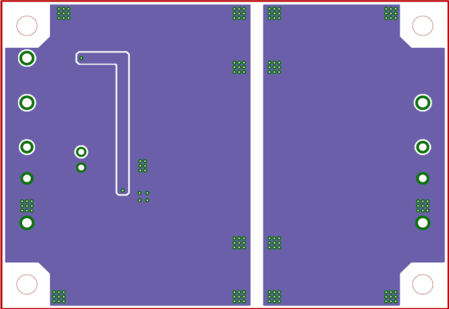
Bottom Side Layer Layout
