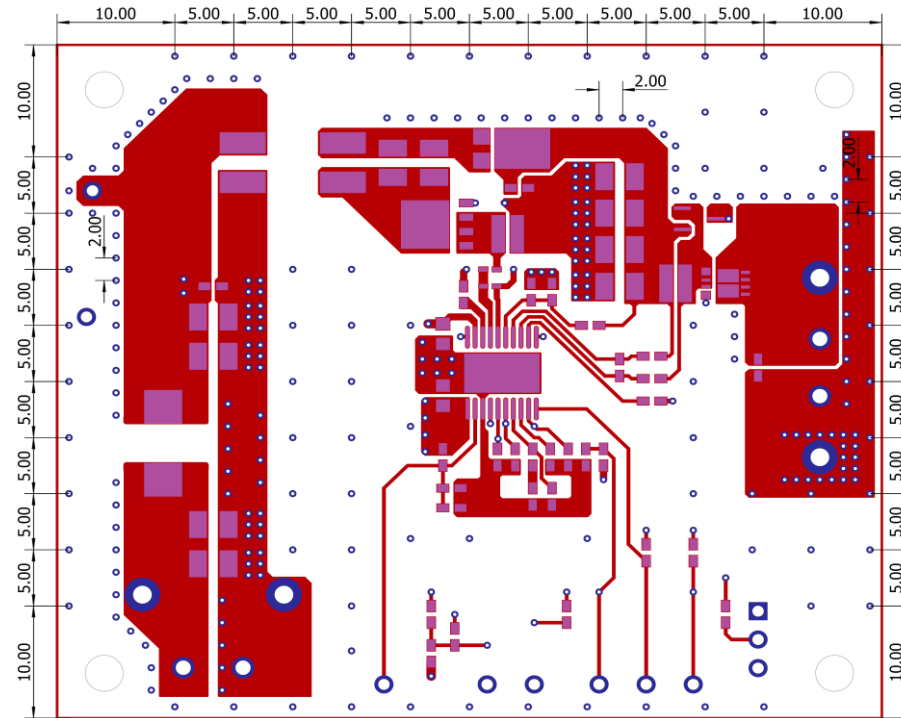
Top layer layout(Top view)
