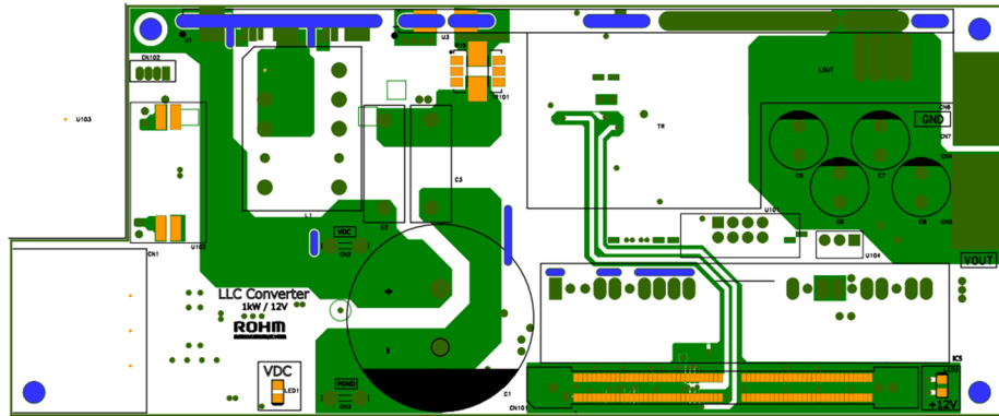
• Top layer
