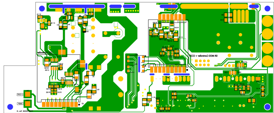
• Botom layer
