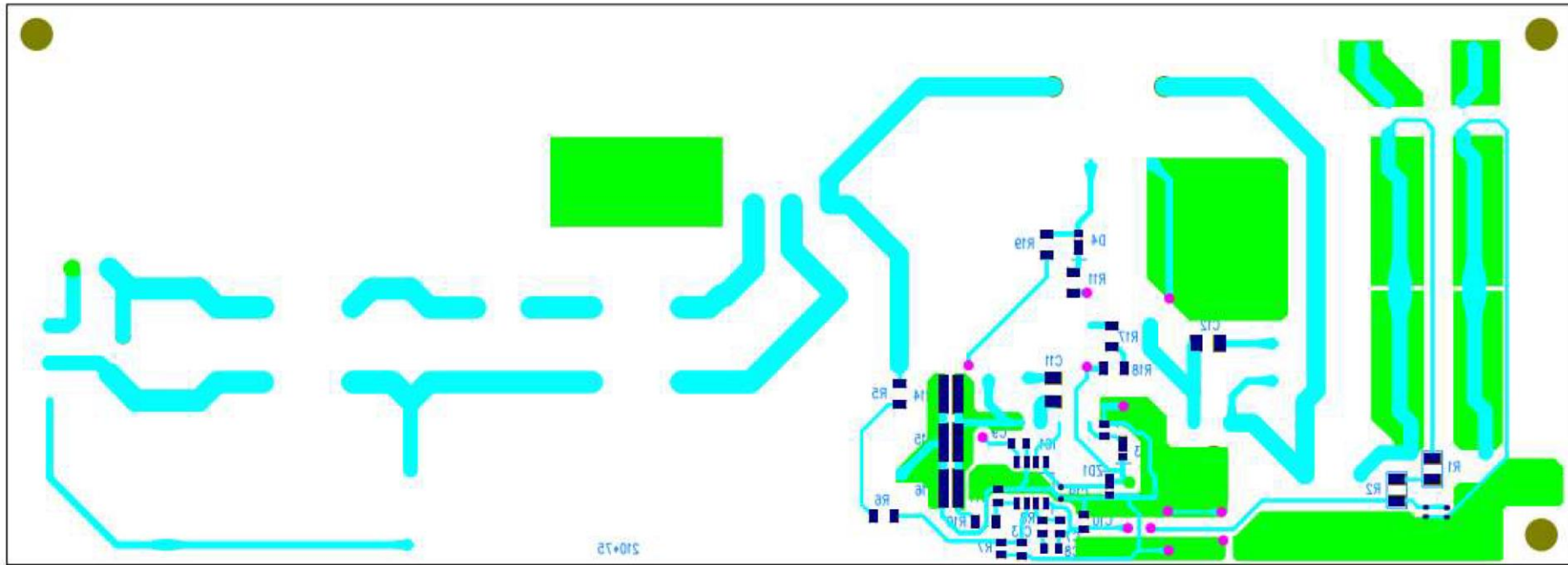
Bottom 側レイアウト (Top view)
