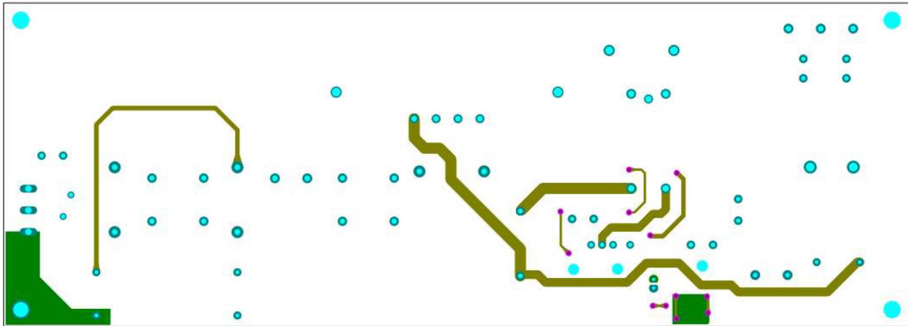
Top 側レイアウト (Top view)
