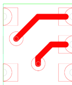
Figure 4. レイアウト(Bottom View)
