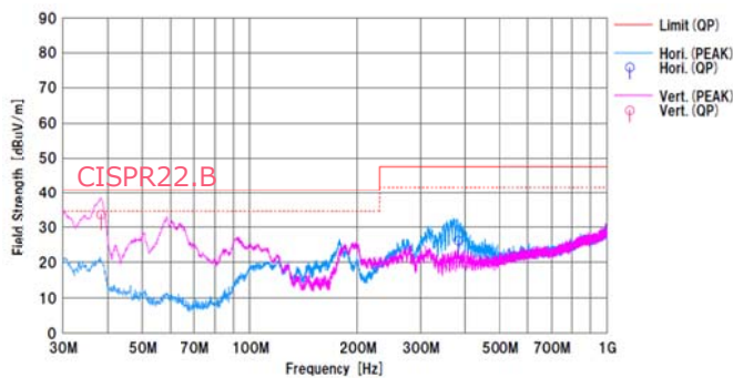
Figure 23. Radiated Emission.1 V IN =110Vac/60Hz, I OUT =0.5A QP margin=6.8dB, AV margin=6.9dB
