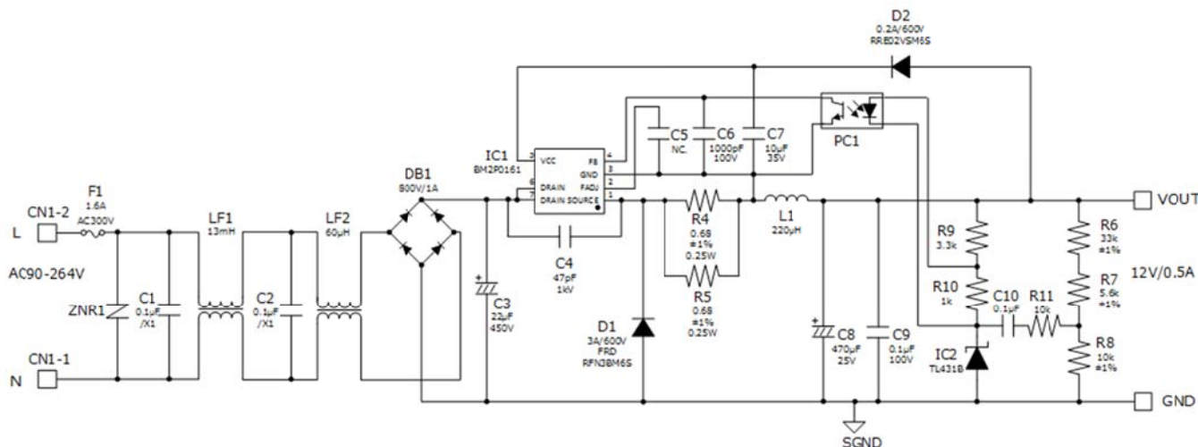
Figure 3. BM2P0161-EVK-002 回路図
