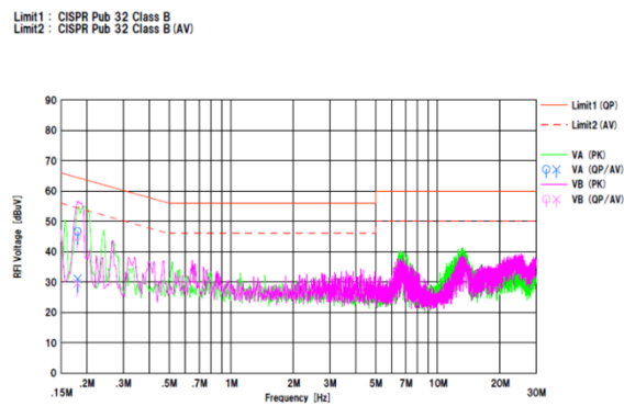
Figure 24. V_{IN} : 115 Vac / 60 Hz, I_{OUT} : 2 A
