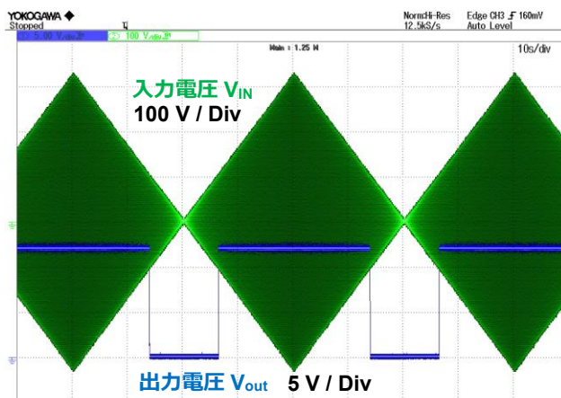
Figure 10. VIN = 0 V から 230V
