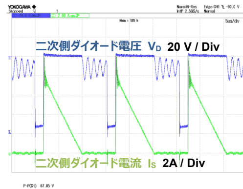
Figure 14. ダイオード波形 V_{IN} = 264 \text{ Vac} , I_{OUT} = 2 \text{ A}
