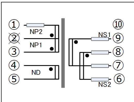
Figure 28. 回路図
