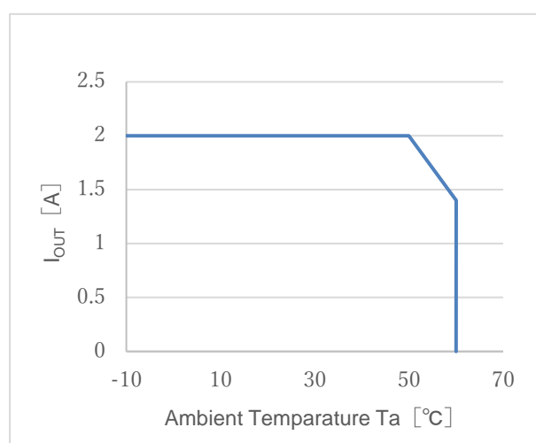
Figure 2. 温度デレレーティングカーブ
