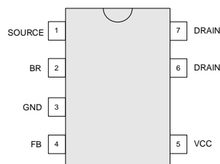
Figure 4. ピン配置図
