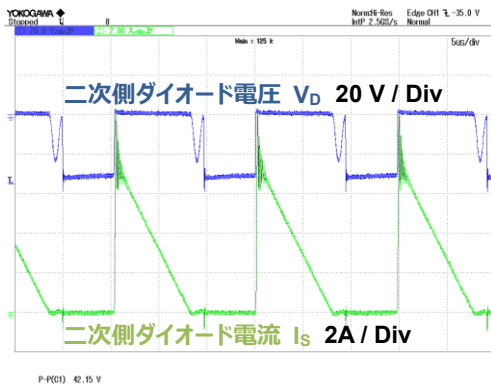
Figure 13. ダイオード波形 V_{IN} = 90 \text{ Vac} , I_{OUT} = 2 \text{ A}
