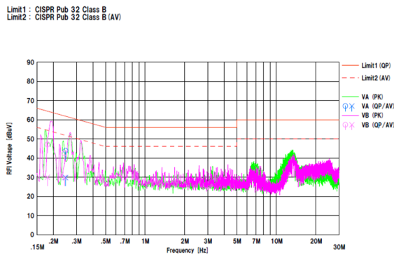
Figure 23. V_{IN} : 230 Vac / 50 Hz, I_{OUT} : 2 A
