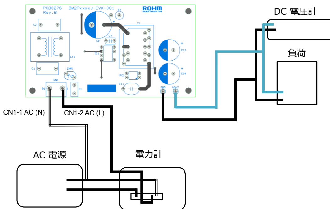
Figure 3. 接続図
