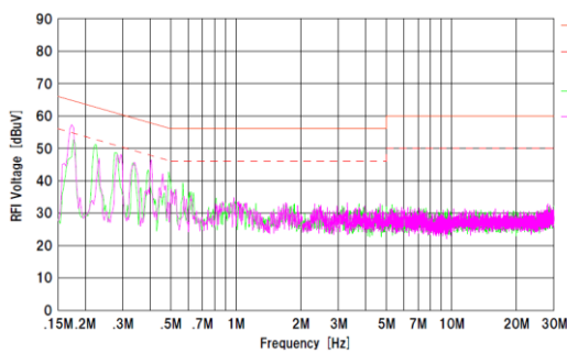
Figure 35. V IN = 110 Vac / 60 Hz, I OUT = 0.75 A QP margin = 17.5 dB, AV margin = 20.8 dB
