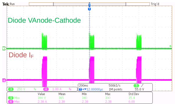
Figure 22. Diode 波形 V_{IN} = 264 \text{ Vac} , 出力短絡
