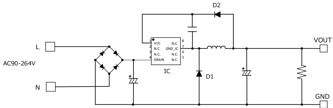
Figure 4. BM2P151X-EVK-001 アプリケーション回路
