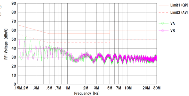
Figure 36. V IN = 230 Vac / 50 Hz, I OUT = 0.75 A QP margin = 23.5 dB, AV margin = 26.5 dB
