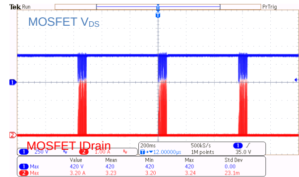
Figure 21. MOSFET 波形 V_{IN} = 264 \text{ Vac} , 出力短絡
