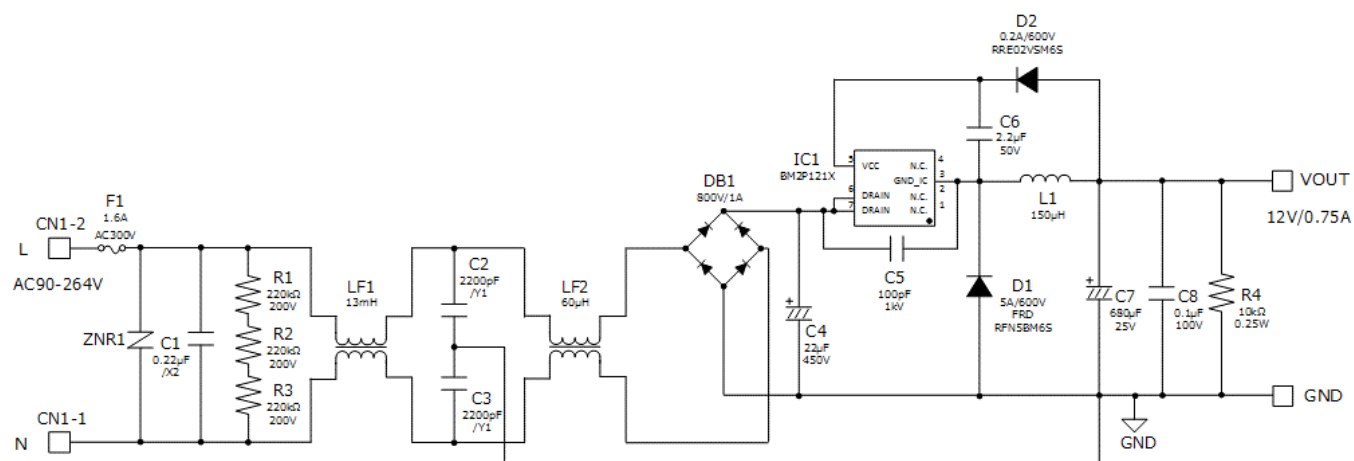
Figure 39. BM2P121X-EVK-001 回路図
