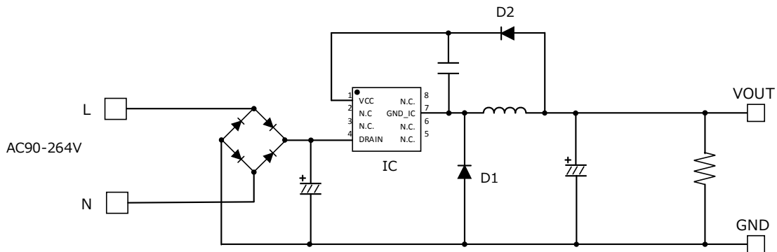
Figure 4. BM2P139TF-EVK-001 アプリケーション回路
