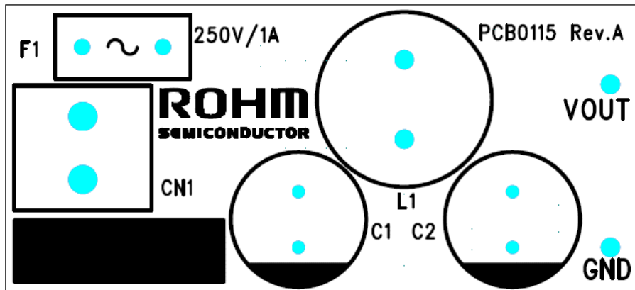
Figure 24. TOP シルksスクリーン (Top view)
