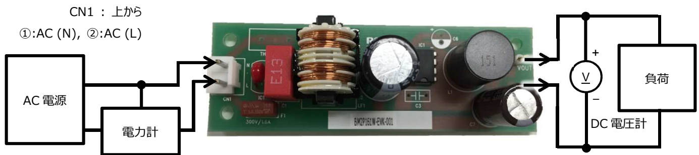
Figure 1. 接続図
