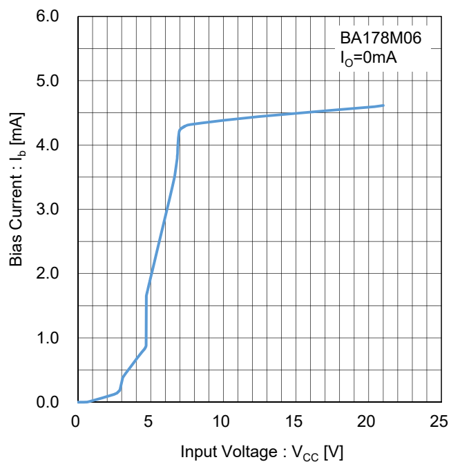
Figure 20. バイアス電流 vs 入力電圧 Test Circuit H
