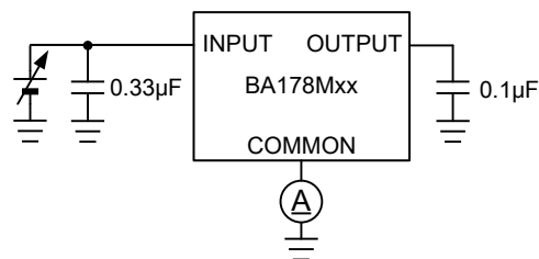
Test Circuit H. バイアス電流 vs 入力電圧
