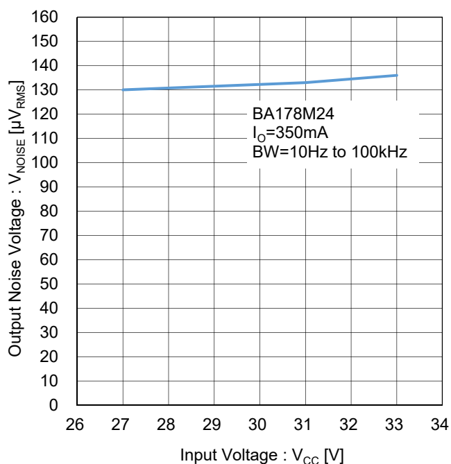
Figure 132. 出力ノイズ電圧 Test Circuit L
