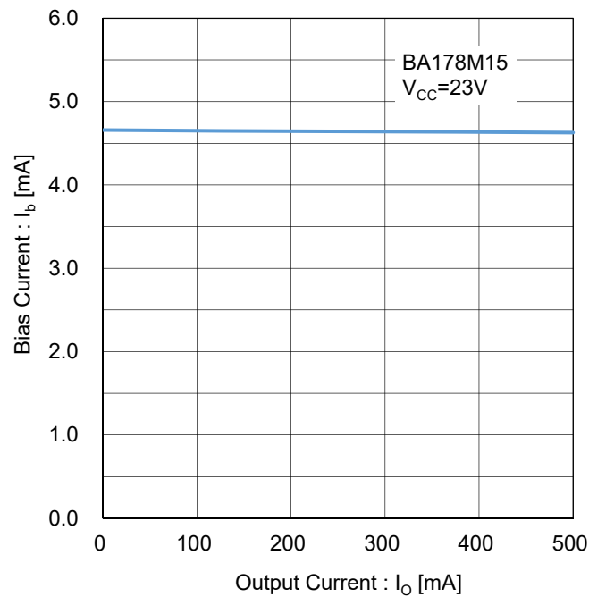
Figure 94. バイアス電流 vs 出力電流 Test Circuit J
