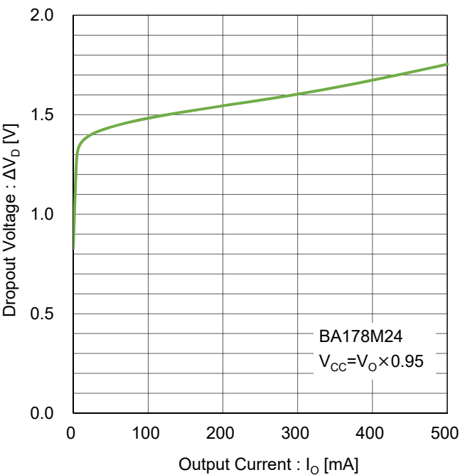
Figure 126. 最小入出力電圧差 vs 出力電流 Test Circuit F
