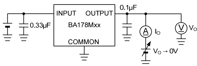
Test Circuit C. 過電流保護
