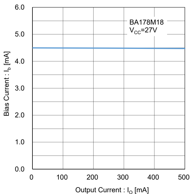
Figure 106. バイアス電流 vs 出力電流 Test Circuit J
