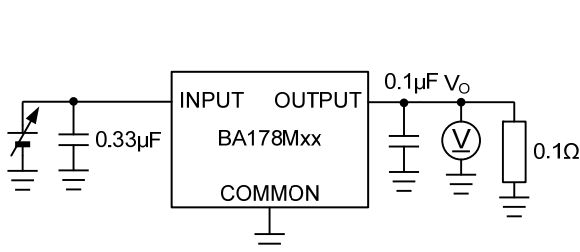
Test Circuit E. 出力短絡電流 vs 入力電圧
