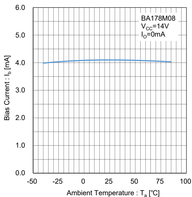
Figure 45. バイアス電流 vs 温度 Test Circuit I
