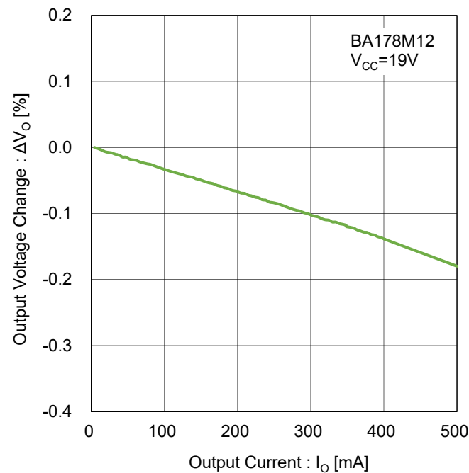
Figure 76. ロードレギュレーション Test Circuit D
