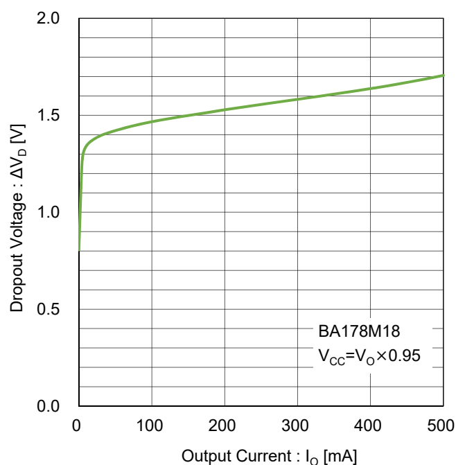
Figure 102. 最小入出力電圧差 vs 出力電流 Test Circuit F
