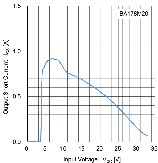
Figure 113. 出力短絡電流 vs 入力電圧 Test Circuit E
