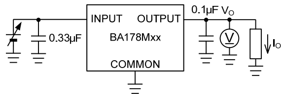
Test Circuit B. ラインレギュレーション
