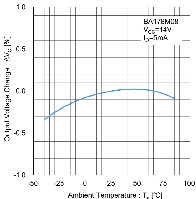
Figure 43. 出力電圧温度安定性 Test Circuit G
