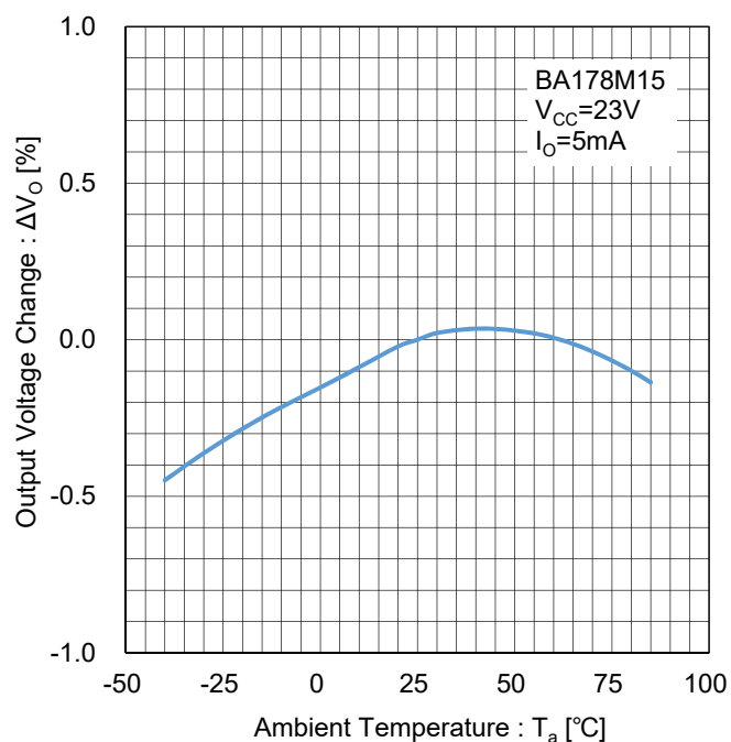
Figure 91. 出力電圧温度安定性 Test Circuit G
