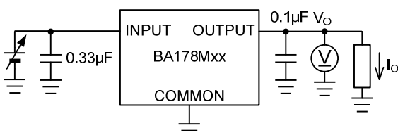
Test Circuit G. 出力電圧温度安定性
