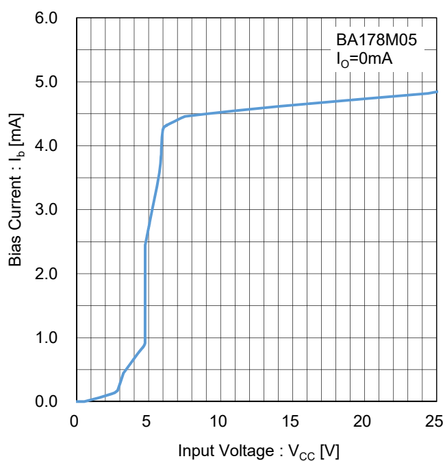
Figure 8. バイアス電流 vs 入力電圧 Test Circuit H
