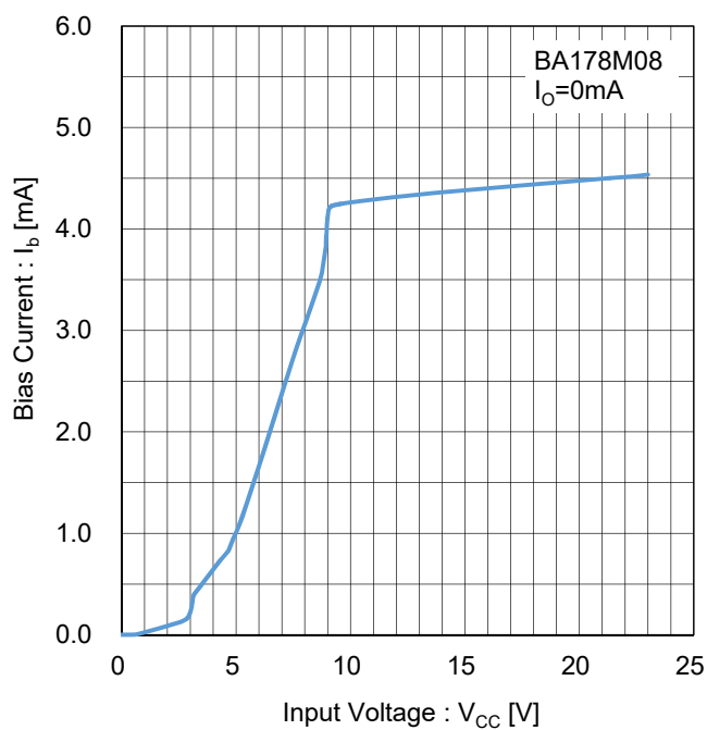
Figure 44. バイアス電流 vs 入力電圧 Test Circuit H
