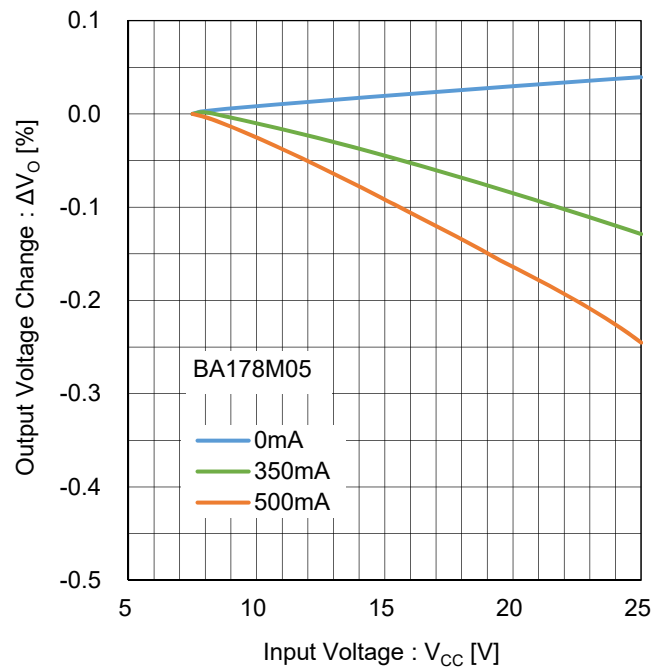
Figure 2. ラインレギュレーション Test Circuit B
