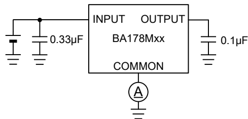
Test Circuit I. バイアス電流 vs 温度
