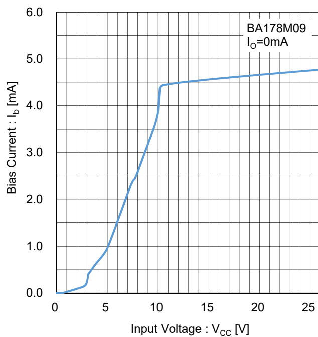
Figure 56. バイアス電流 vs 入力電圧 Test Circuit H
