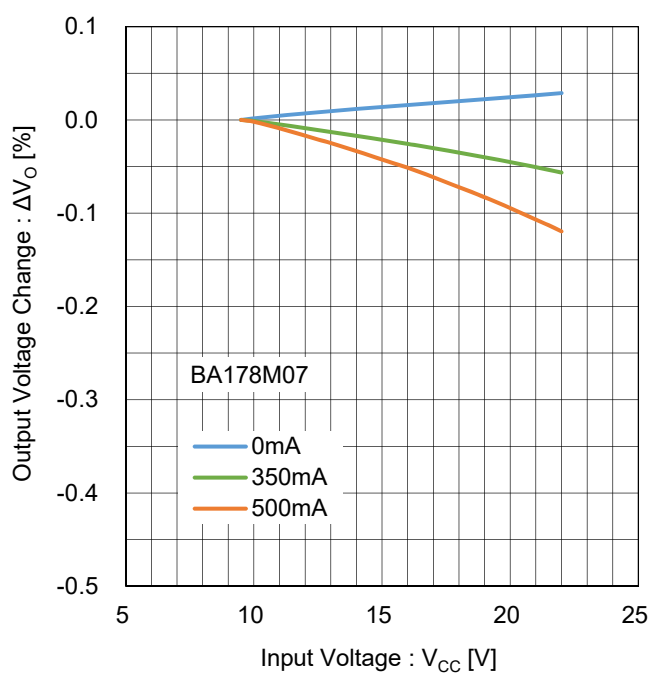
Figure 26. ラインレギュレーション Test Circuit B
