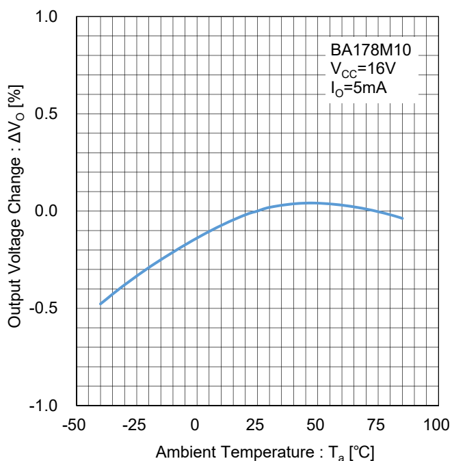
Figure 67. 出力電圧温度安定性 Test Circuit G
