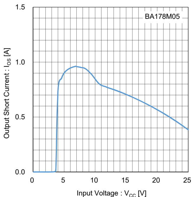
Figure 5. 出力短絡電流 vs 入力電圧 Test Circuit E
