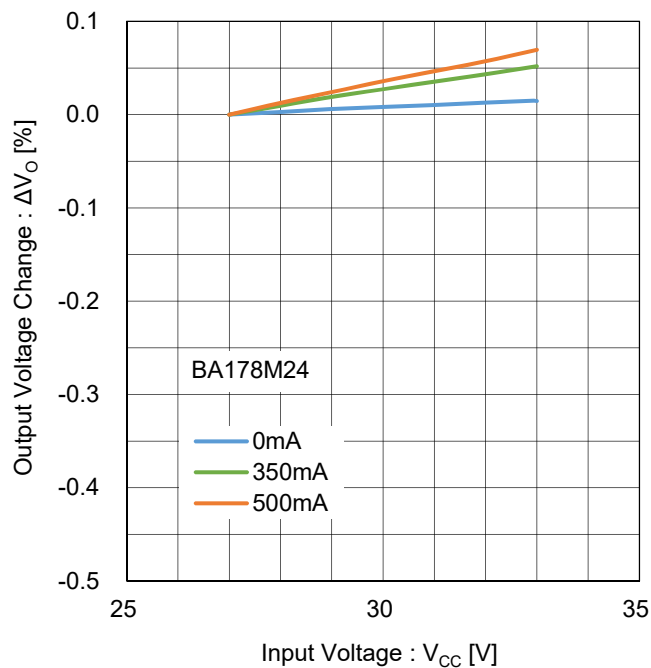
Figure 122. ラインレギュレーション Test Circuit B
