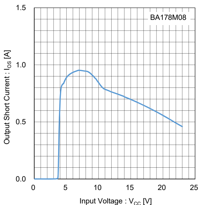
Figure 41. 出力短絡電流 vs 入力電圧 Test Circuit E
