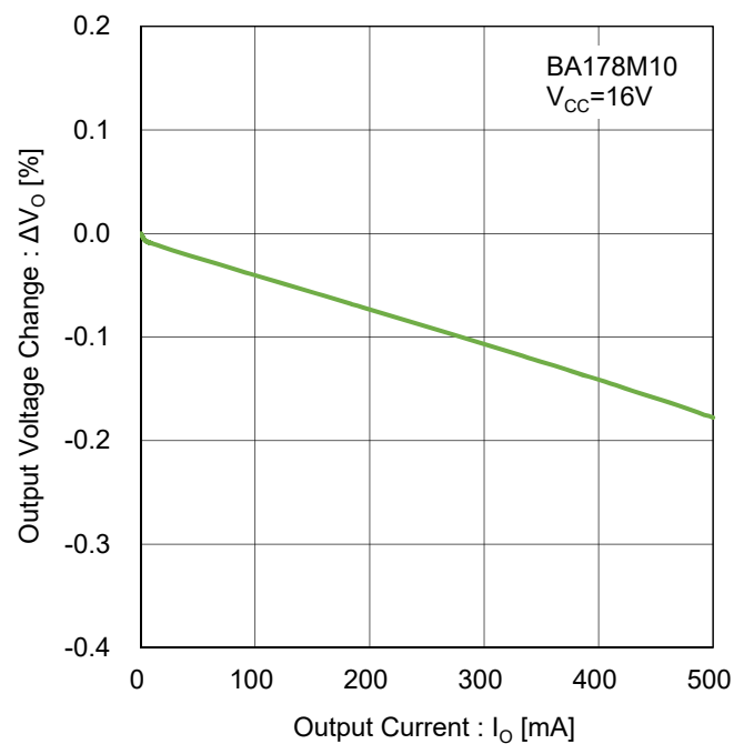
Figure 64. ロードレギュレーション Test Circuit D
