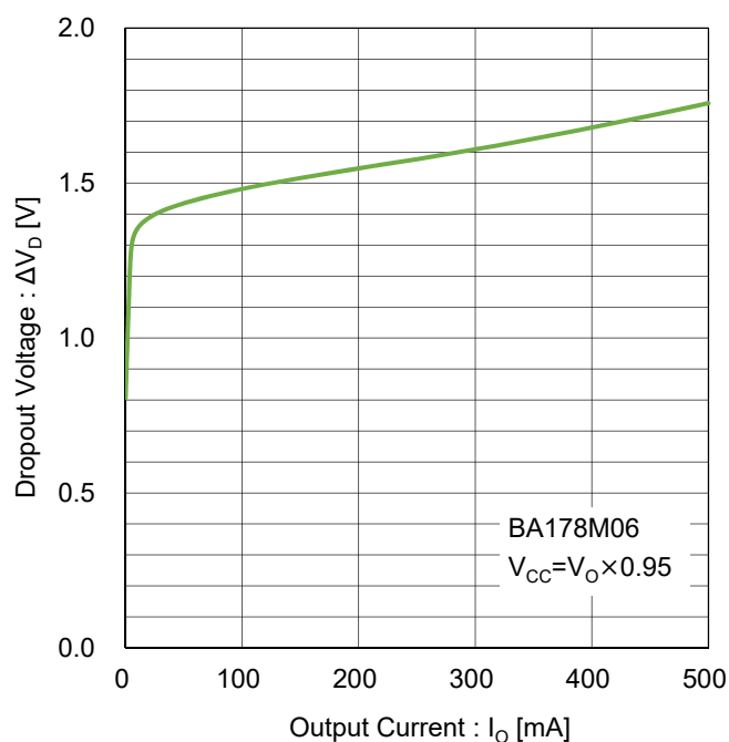
Figure 18. 最小入出力電圧差 vs 出力電流 Test Circuit F
