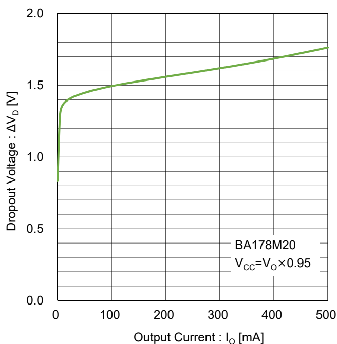
Figure 114. 最小入出力電圧差 vs 出力電流 Test Circuit F
