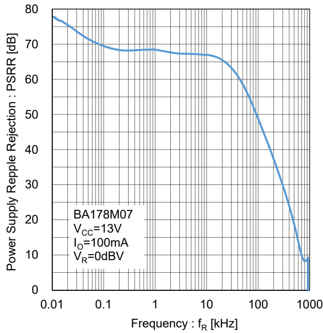
Figure 35. リップルリジェクション Test Circuit K
