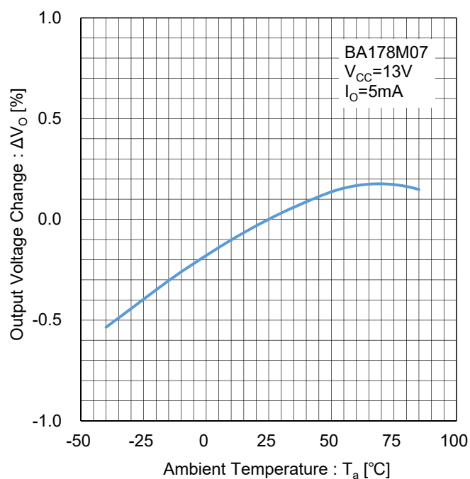
Figure 31. 出力電圧温度安定性 Test Circuit G
