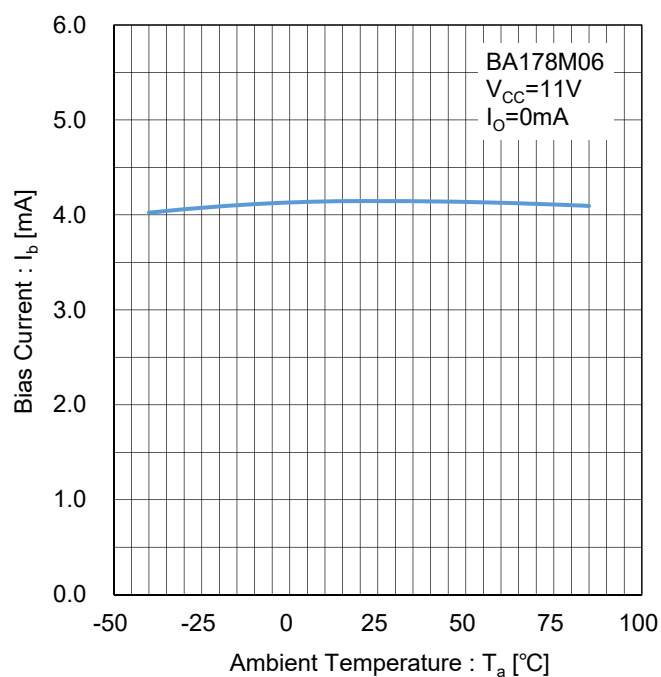
Figure 21. バイアス電流 vs 温度 Test Circuit I
