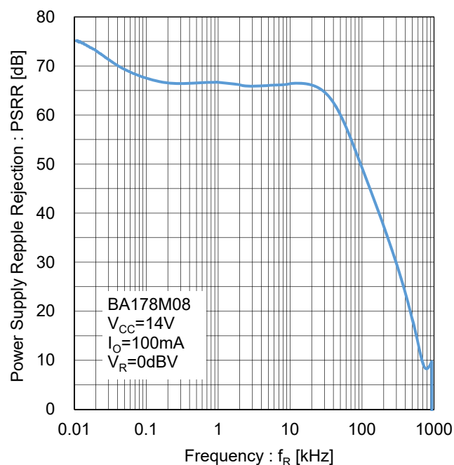
Figure 47. リップルリジェクション Test Circuit K
