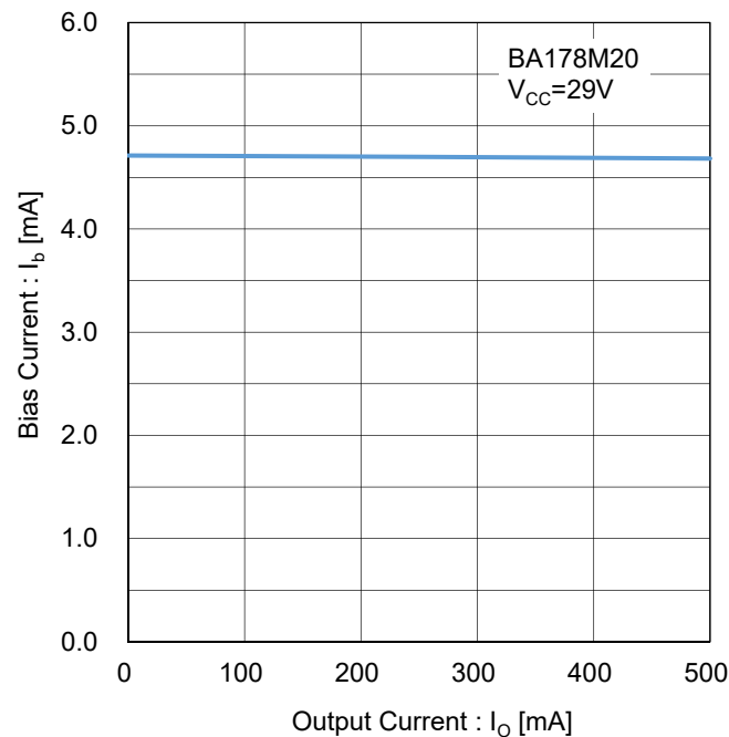
Figure 118. バイアス電流 vs 出力電流 Test Circuit J
