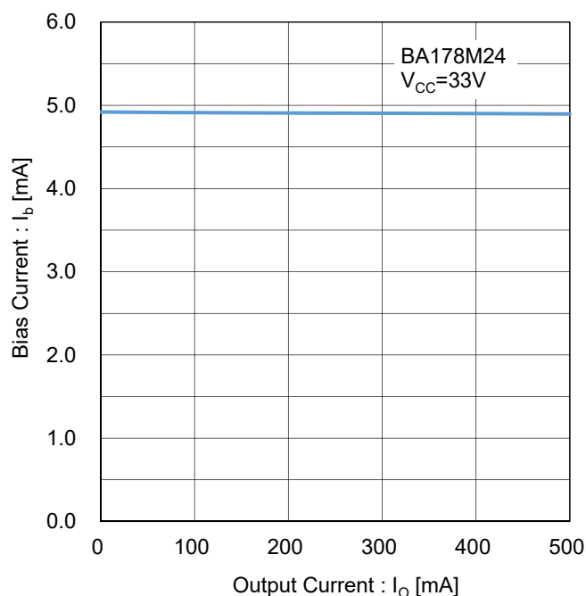
Figure 130. バイアス電流 vs 出力電流 Test Circuit J
