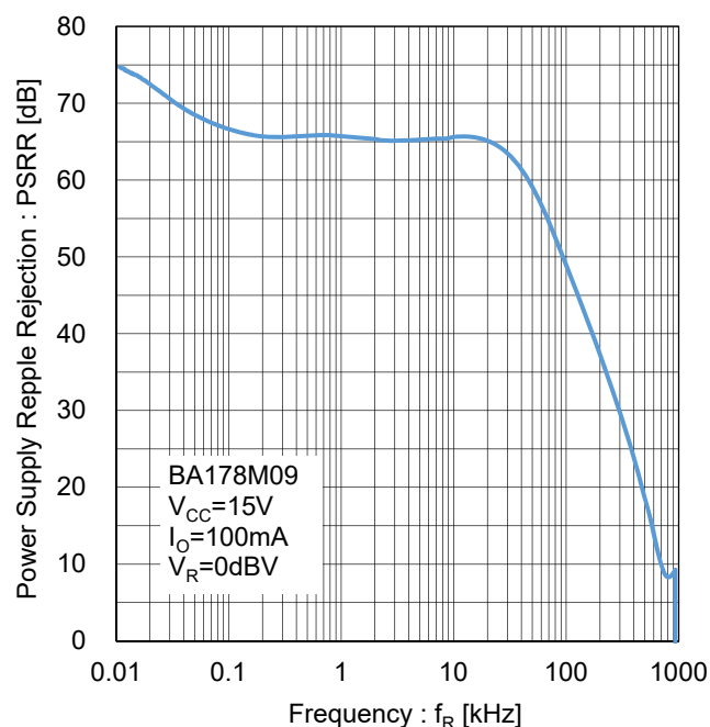
Figure 59. リップルリジェクション Test Circuit K
