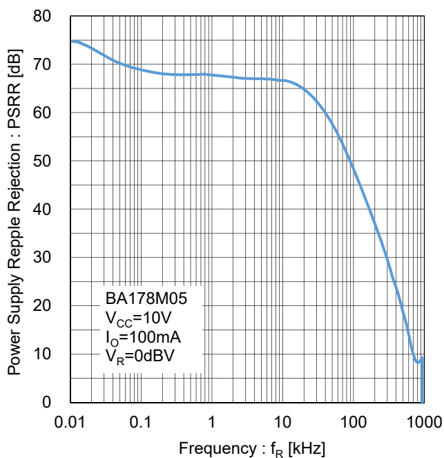
Figure 11. リップルリジェクション Test Circuit K
