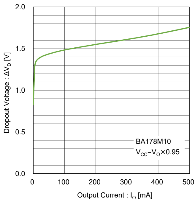
Figure 66. 最小入出力電圧差 vs 出力電流 Test Circuit F
