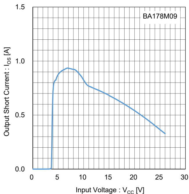
Figure 53. 出力短絡電流 vs 入力電圧 Test Circuit E
