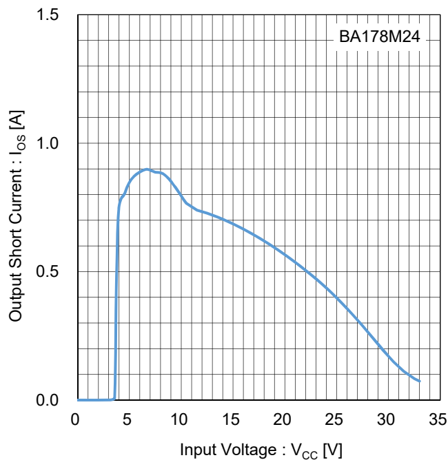
Figure 125. 出力短絡電流 vs 入力電圧 Test Circuit E
