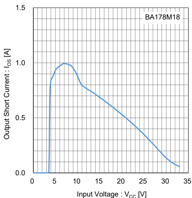
Figure 101. 出力短絡電流 vs 入力電圧 Test Circuit E
