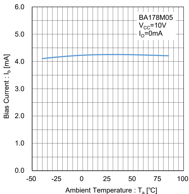
Figure 9. バイアス電流 vs 温度 Test Circuit I
