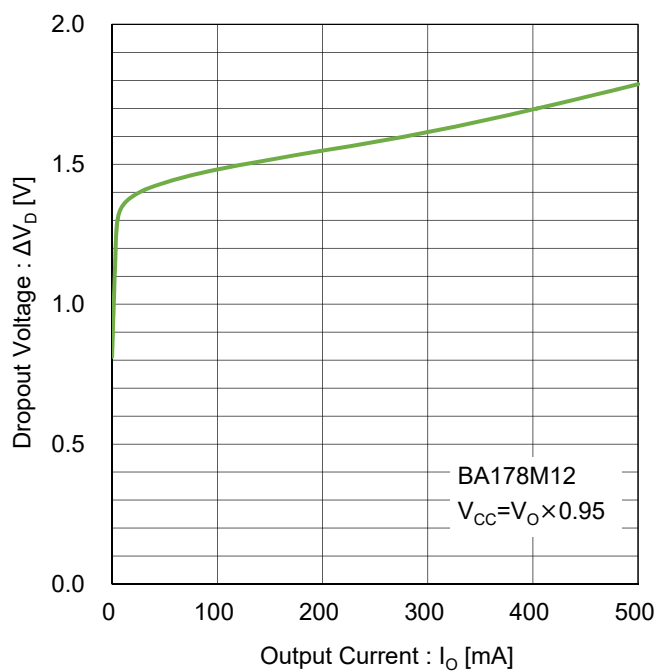
Figure 78. 最小入出力電圧差 vs 出力電流 Test Circuit F
