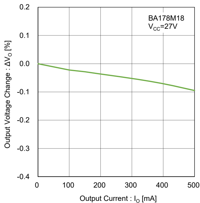
Figure 100. ロードレギュレーション Test Circuit D
