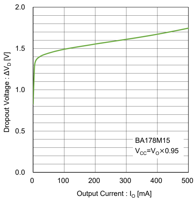
Figure 90. 最小入出力電圧差 vs 出力電流 Test Circuit F
