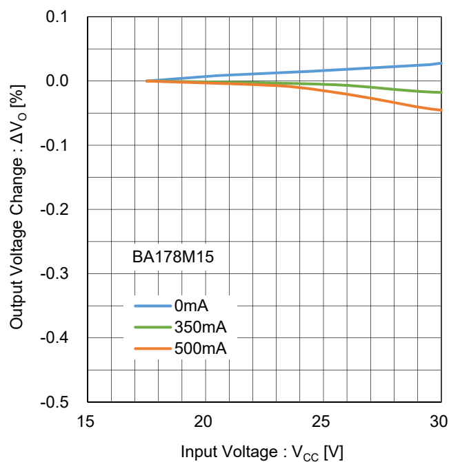
Figure 86. ラインレギュレーション Test Circuit B
