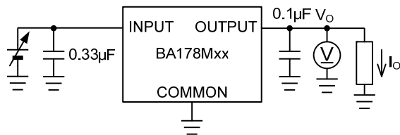
Test Circuit A. 出力電圧 vs 入力電圧
