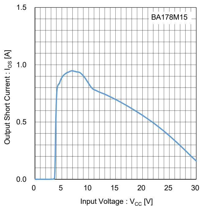
Figure 89. 出力短絡電流 vs 入力電圧 Test Circuit E
