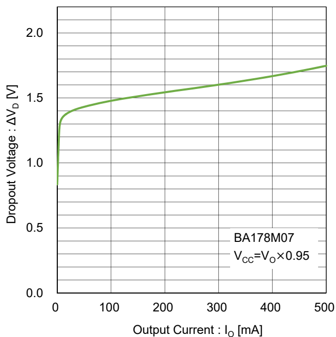
Figure 30. 最小入出力電圧差 vs 出力電流 Test Circuit F
