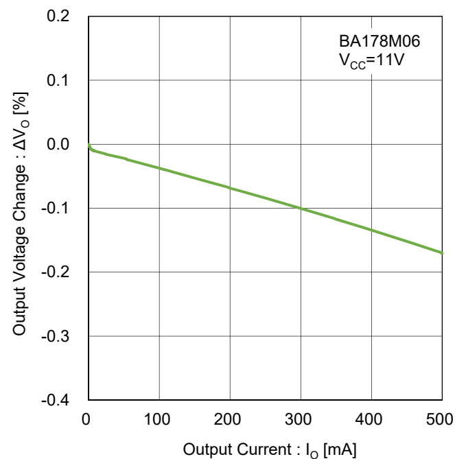
Figure 16. ロードレギュレーション Test Circuit D
