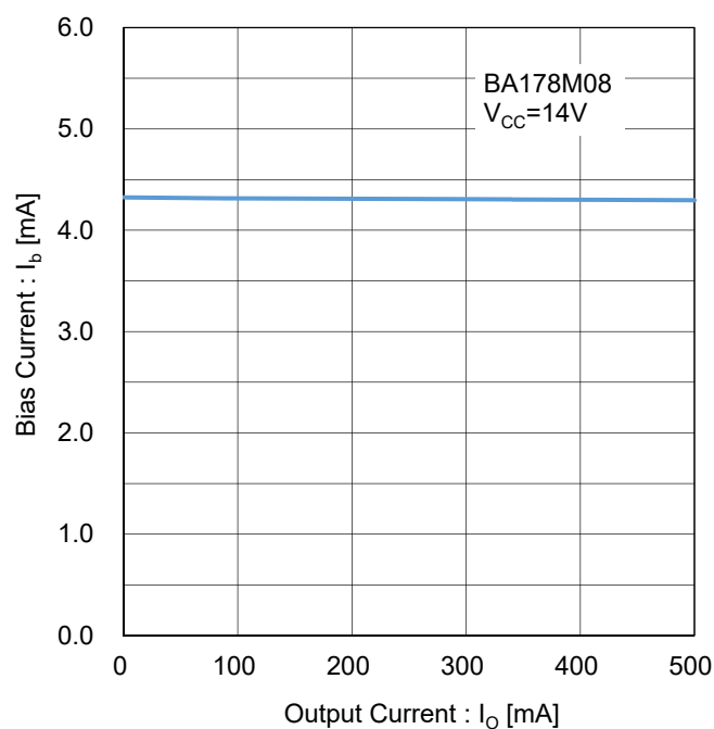
Figure 46. バイアス電流 vs 出力電流 Test Circuit J
