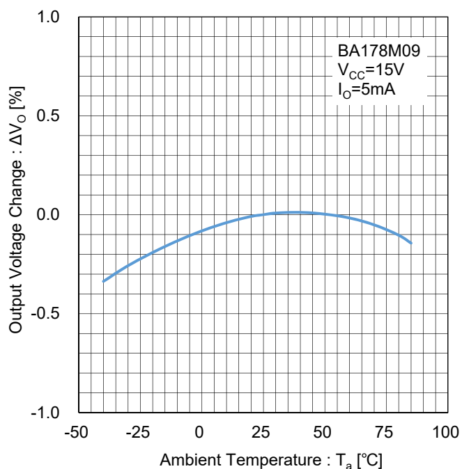
Figure 55. 出力電圧温度安定性 Test Circuit G
