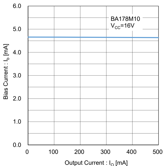
Figure 70. バイアス電流 vs 出力電流 Test Circuit J
