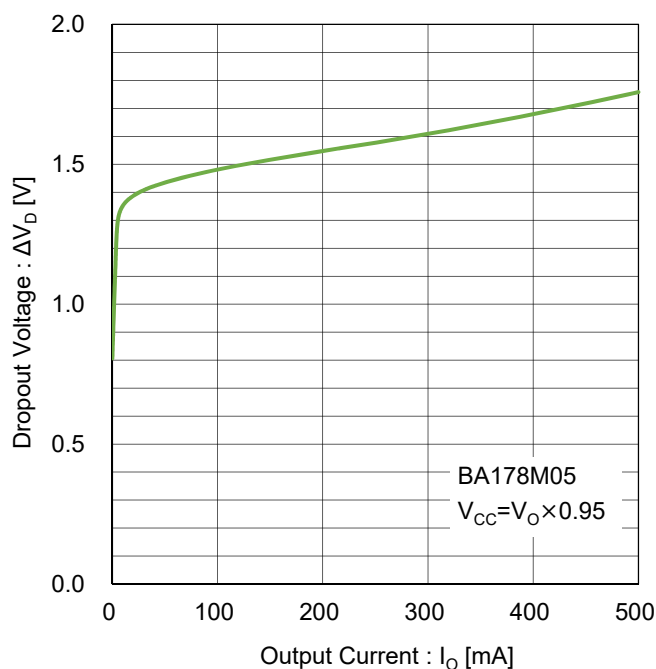
Figure 6. 最小入出力電圧差 vs 出力電流 Test Circuit F
