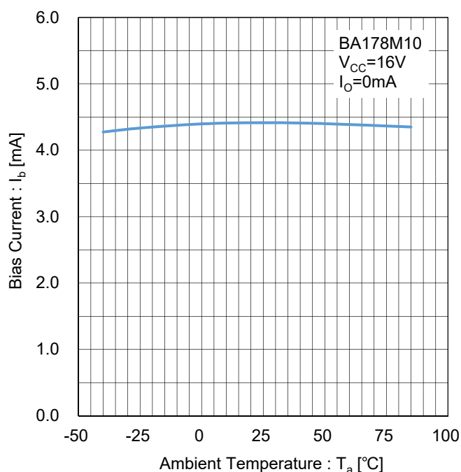
Figure 69. バイアス電流 vs 温度 Test Circuit I
