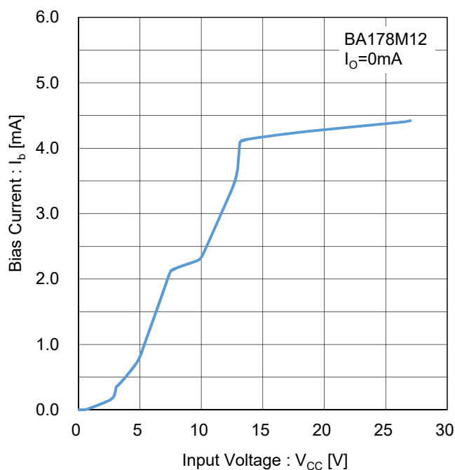
Figure 80. バイアス電流 vs 入力電圧 Test Circuit H
