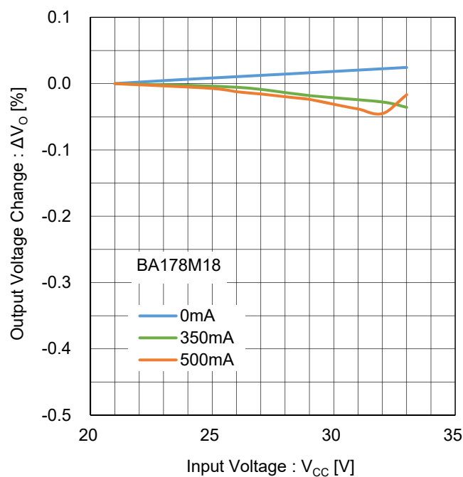
Figure 98. ラインレギュレーション Test Circuit B
