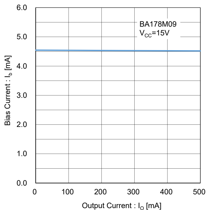
Figure 58. バイアス電流 vs 出力電流 Test Circuit J
