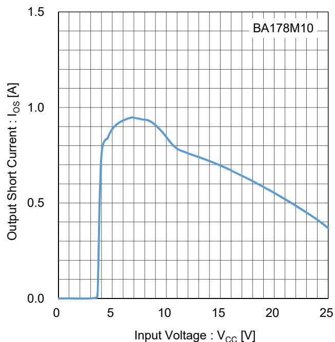
Figure 65. 出力短絡電流 vs 入力電圧 Test Circuit E
