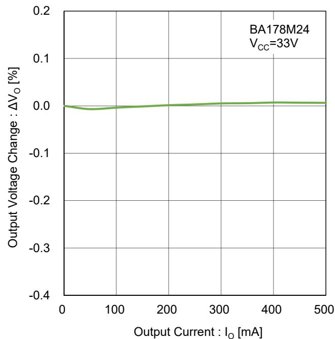
Figure 124. ロードレギュレーション Test Circuit D
