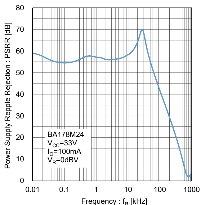
Figure 131. リップルリジェクション Test Circuit K
