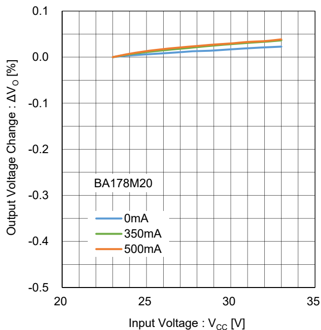
Figure 110. ラインレギュレーション Test Circuit B
