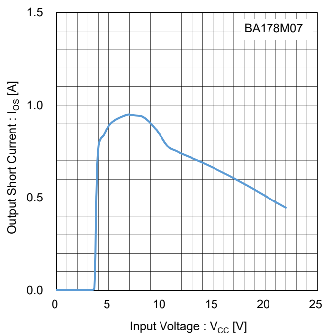
Figure 29. 出力短絡電流 vs 入力電圧 Test Circuit E
