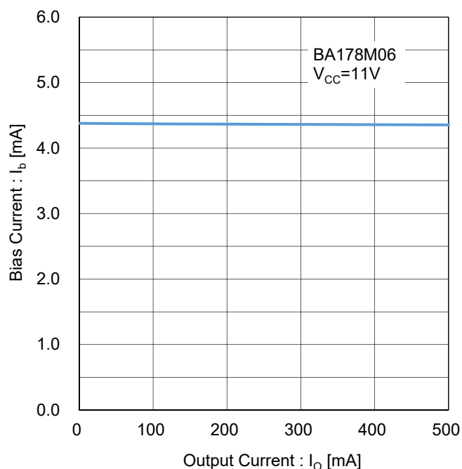
Figure 22. バイアス電流 vs 出力電流 Test Circuit J
