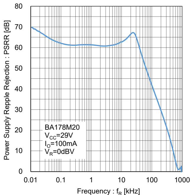
Figure 119. リップルリジェクション Test Circuit K
