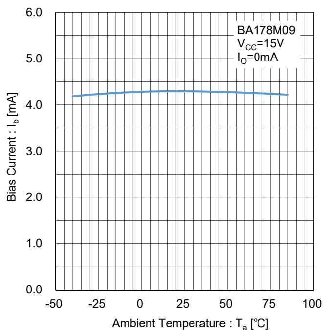
Figure 57. バイアス電流 vs 温度 Test Circuit I
