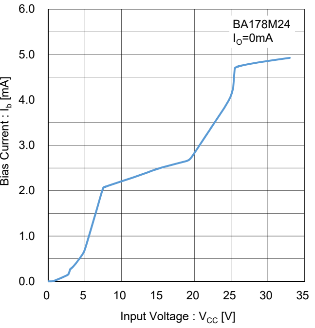
Figure 128. バイアス電流 vs 入力電圧 Test Circuit H
