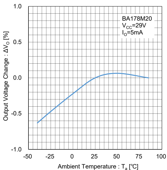
Figure 115. 出力電圧温度安定性 Test Circuit G
