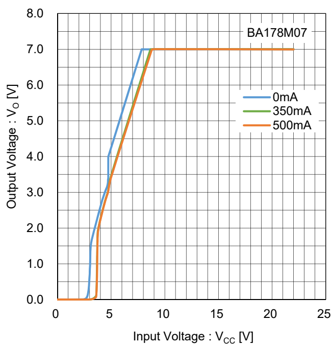
Figure 25. 出力電圧 vs 入力電圧 Test Circuit A
