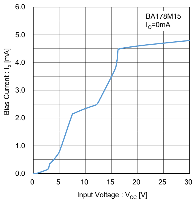
Figure 92. バイアス電流 vs 入力電圧 Test Circuit H
