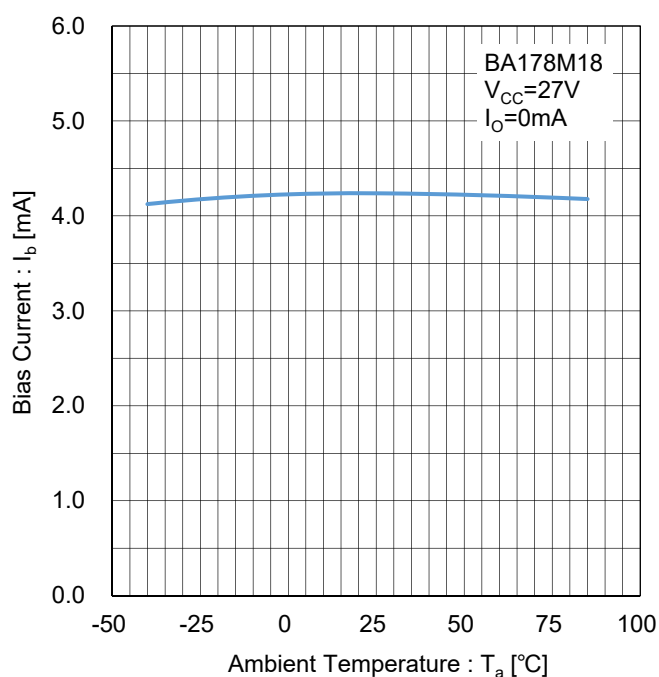
Figure 105. バイアス電流 vs 温度 Test Circuit I
