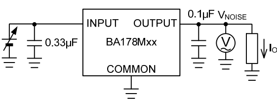
Test Circuit L. 出力ノイズ電圧
