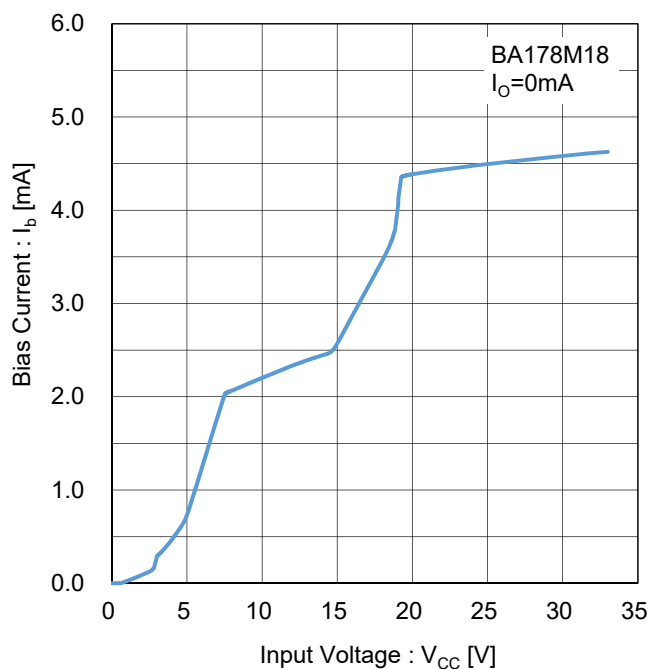
Figure 104. バイアス電流 vs 入力電圧 Test Circuit H
