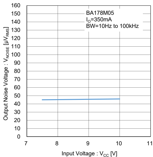
Figure 12. 出力ノイズ電圧 Test Circuit L
