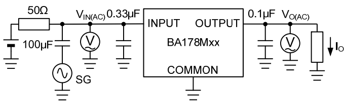
Test Circuit K. リプルリジェクション
