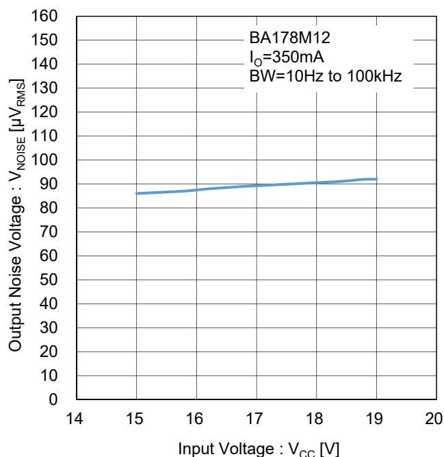
Figure 84. 出力ノイズ電圧 Test Circuit L
