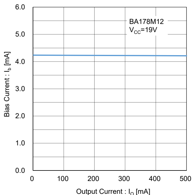
Figure 82. バイアス電流 vs 出力電流 Test Circuit J
