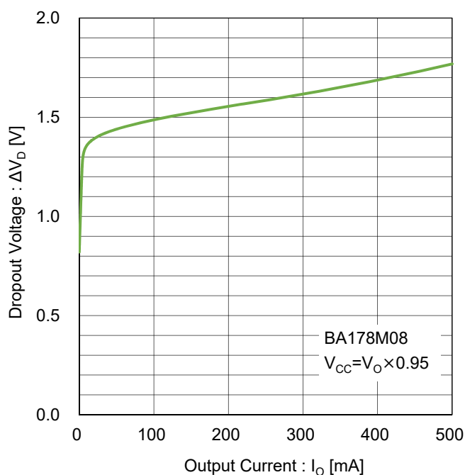
Figure 42. 最小入出力電圧差 vs 出力電流 Test Circuit F
