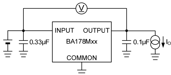
Test Circuit F. 最小入出力電圧差 vs 出力電流
