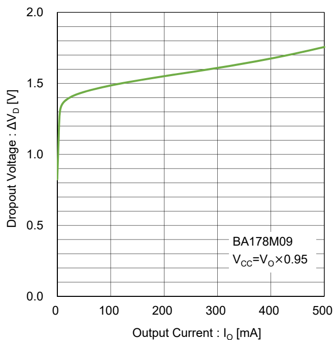
Figure 54. 最小入出力電圧差 vs 出力電流 Test Circuit F
