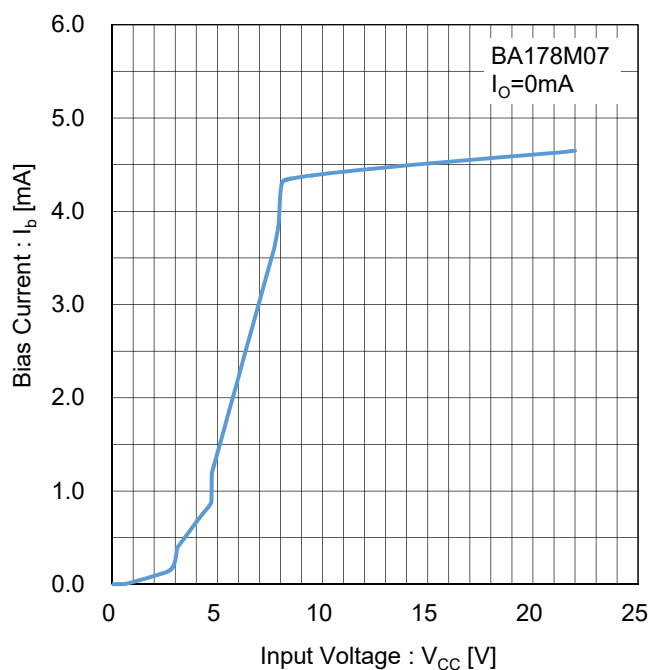
Figure 32. バイアス電流 vs 入力電圧 Test Circuit H
