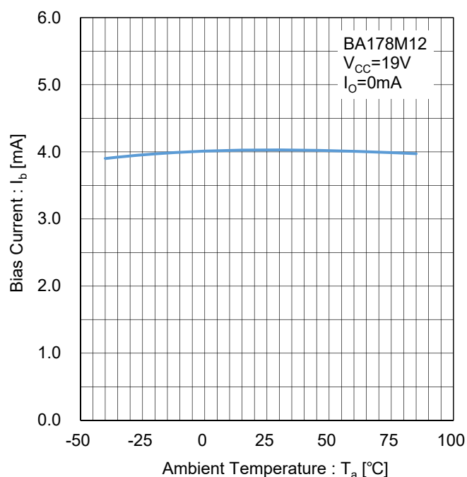
Figure 81. バイアス電流 vs 温度 Test Circuit I
