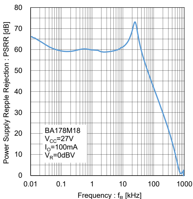
Figure 107. リップルリジェクション Test Circuit K
