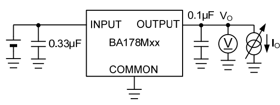
Test Circuit D. ロードレギュレーション
