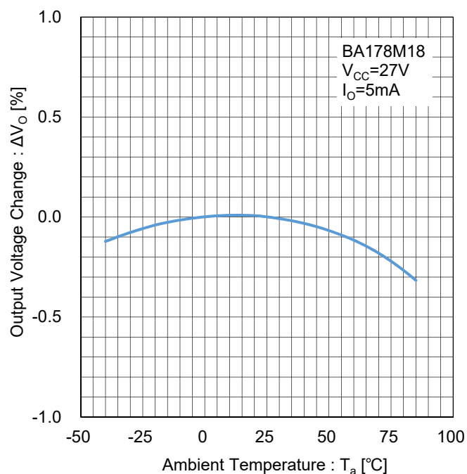
Figure 103. 出力電圧温度安定性 Test Circuit G
