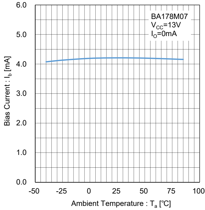
Figure 33. バイアス電流 vs 温度 Test Circuit I
