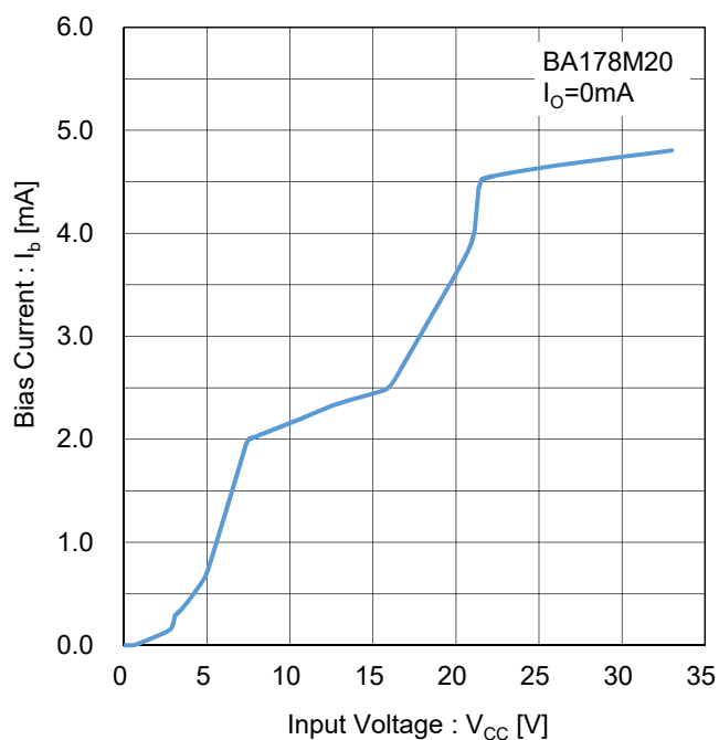
Figure 116. バイアス電流 vs 入力電圧 Test Circuit H
