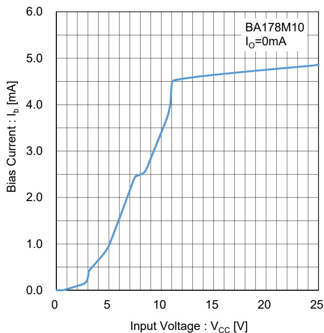
Figure 68. バイアス電流 vs 入力電圧 Test Circuit H
