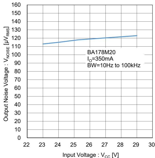
Figure 120. 出力ノイズ電圧 Test Circuit L
