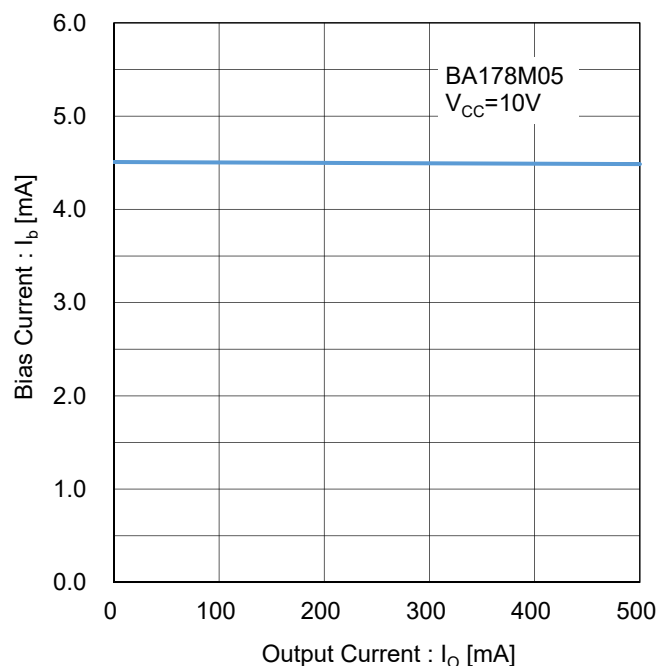
Figure 10. バイアス電流 vs 出力電流 Test Circuit J
