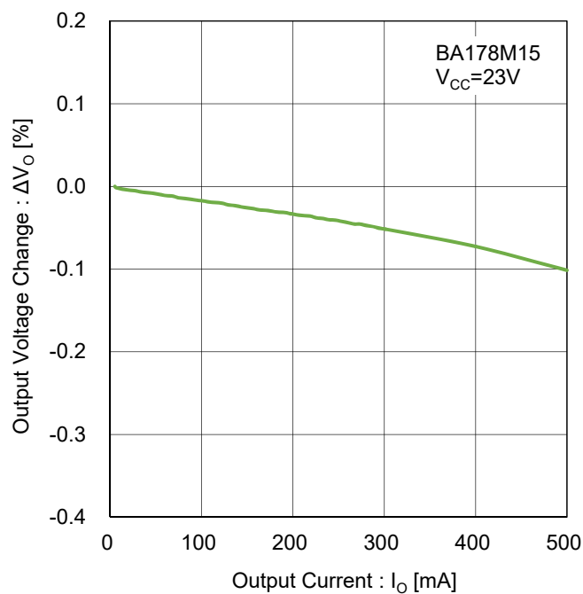
Figure 88. ロードレギュレーション Test Circuit D
