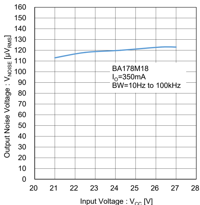
Figure 108. 出力ノイズ電圧 Test Circuit L
