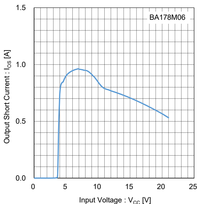
Figure 17. 出力短絡電流 vs 入力電圧 Test Circuit E
