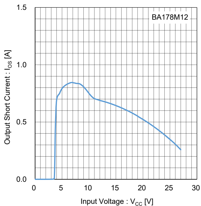
Figure 77. 出力短絡電流 vs 入力電圧 Test Circuit E
