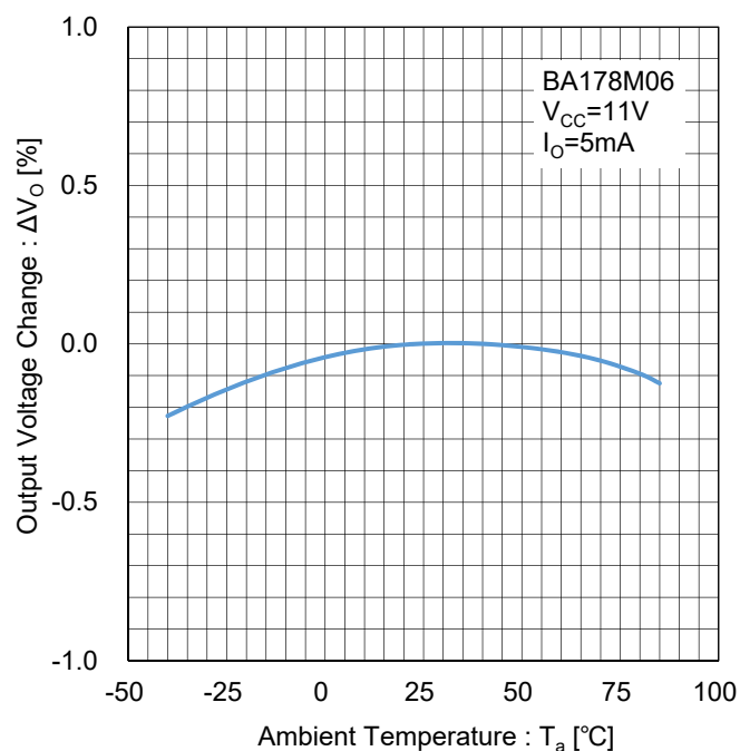
Figure 19. 出力電圧温度安定性 Test Circuit G
