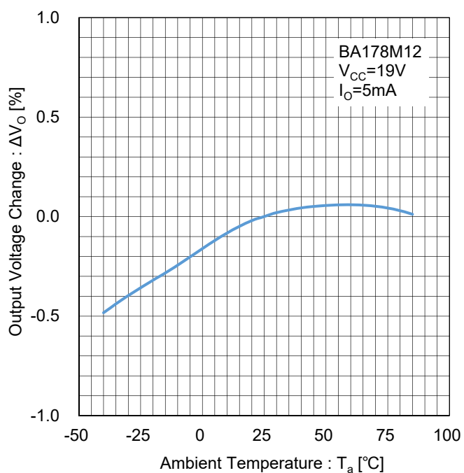
Figure 79. 出力電圧温度安定性 Test Circuit G
