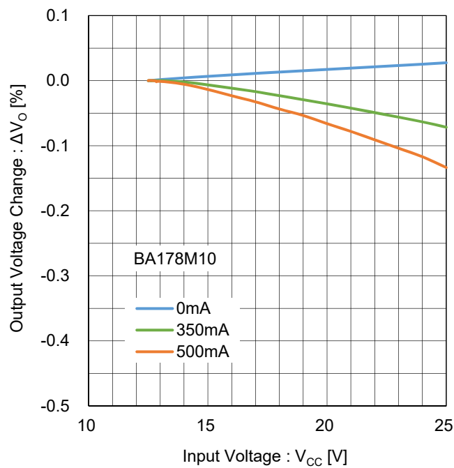
Figure 62. ラインレギュレーション Test Circuit B
