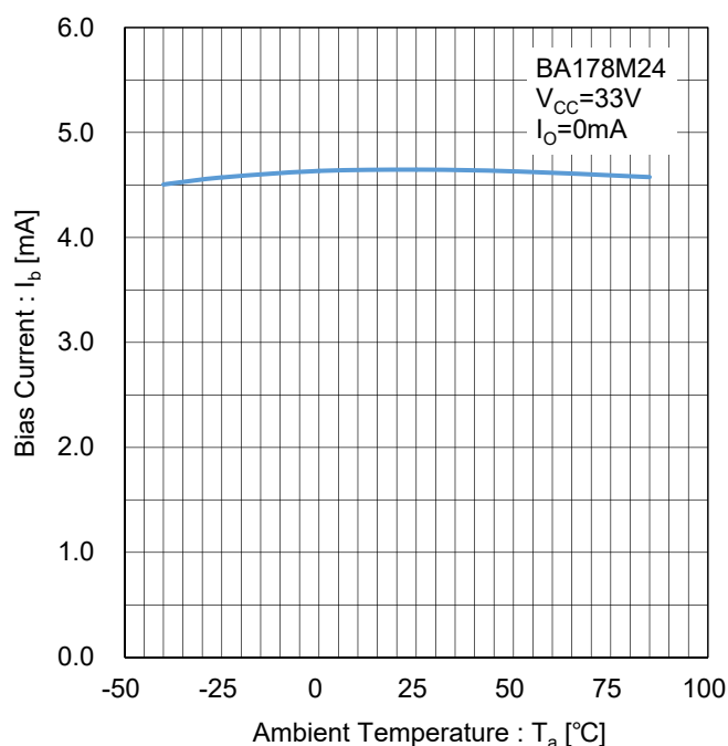
Figure 129. バイアス電流 vs 温度 Test Circuit I
