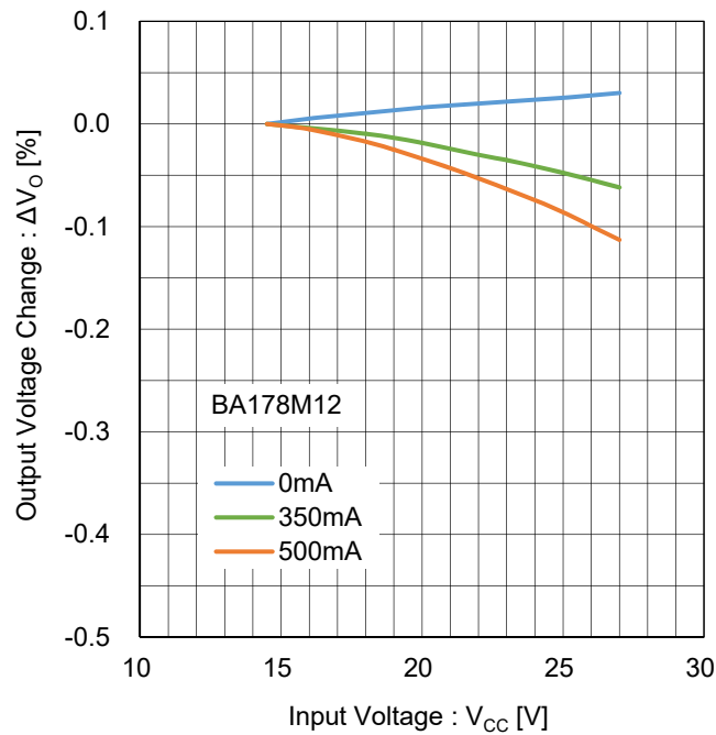
Figure 74. ラインレギュレーション Test Circuit B
