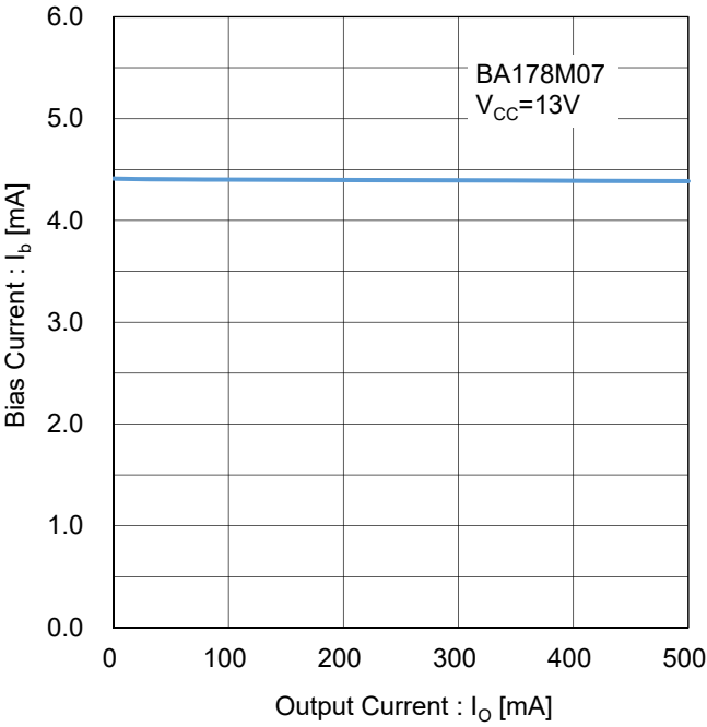
Figure 34. バイアス電流 vs 出力電流 Test Circuit J
