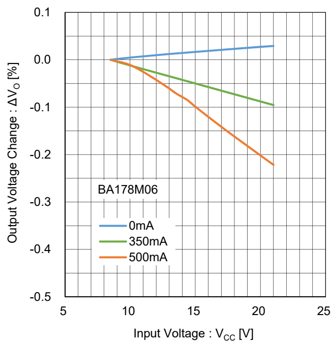
Figure 14. ラインレギュレーション Test Circuit B
