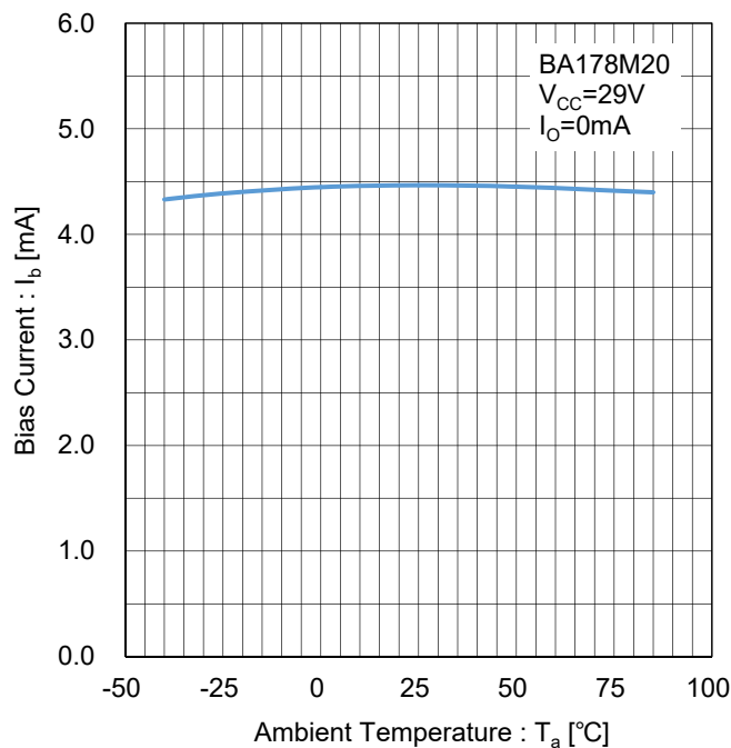
Figure 117. バイアス電流 vs 温度 Test Circuit I
