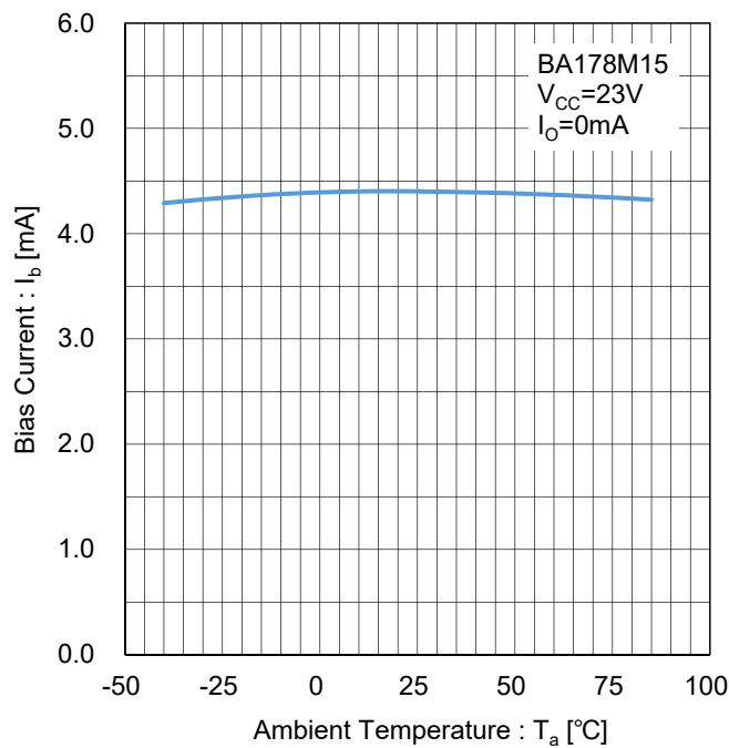
Figure 93. バイアス電流 vs 温度 Test Circuit I
