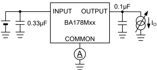
Test Circuit J. バイアス電流 vs 出力電流
