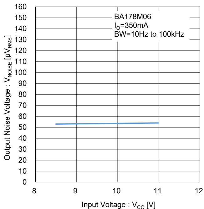
Figure 24. 出力ノイズ電圧 Test Circuit L
