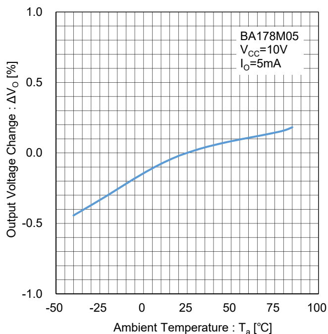
Figure 7. 出力電圧温度安定性 Test Circuit G
