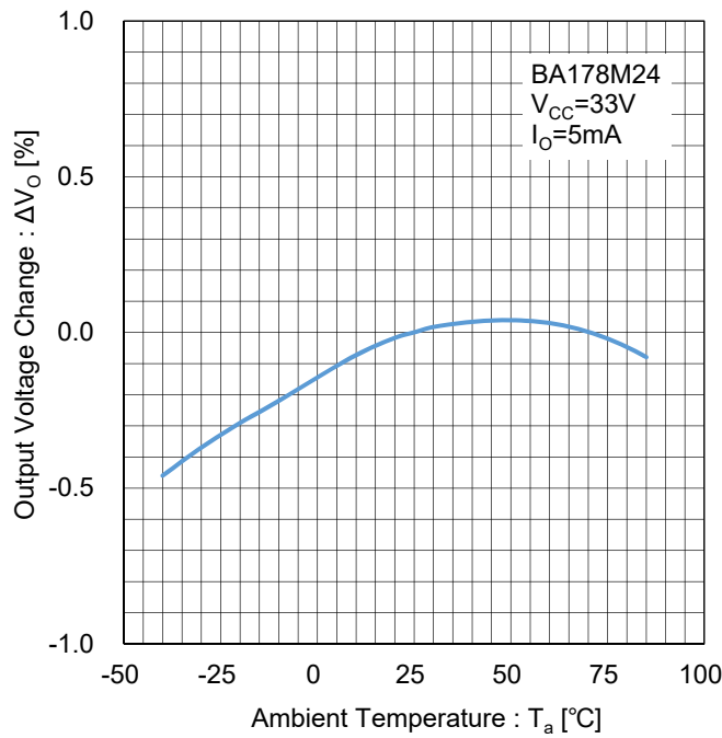
Figure 127. 出力電圧温度安定性 Test Circuit G
