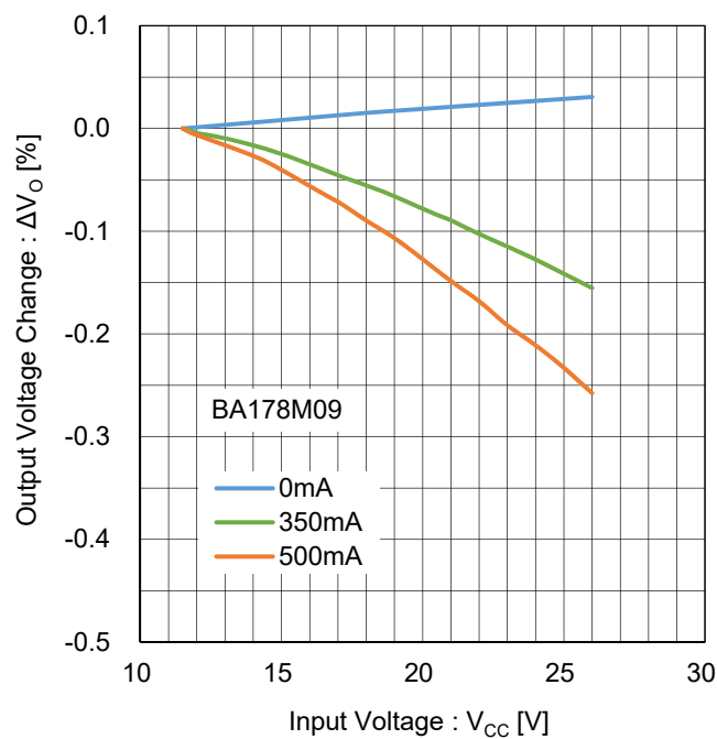
Figure 50. ラインレギュレーション Test Circuit B
