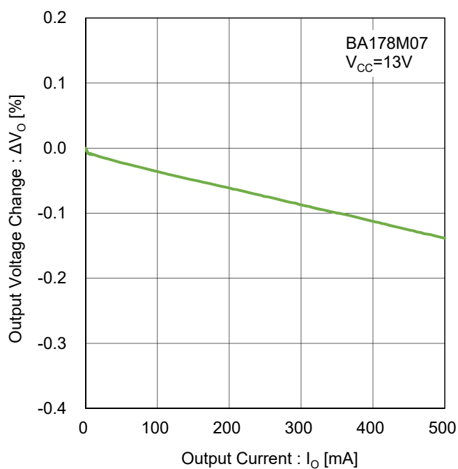
Figure 28. ロードレギュレーション Test Circuit D
