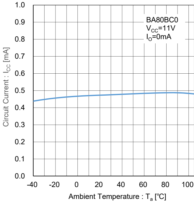
Figure 131. 回路電流 vs 温度 Test Circuit I
