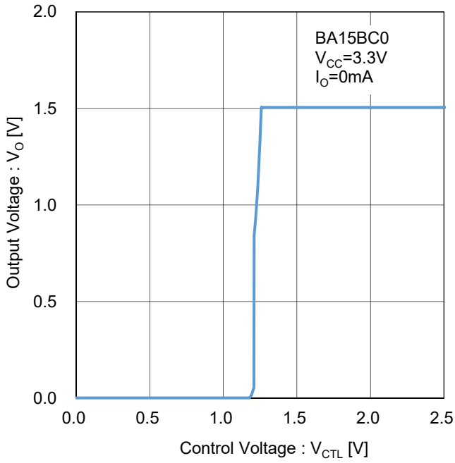
Figure 13. 出力電圧 vs CTL ピン電圧 Test Circuit K
