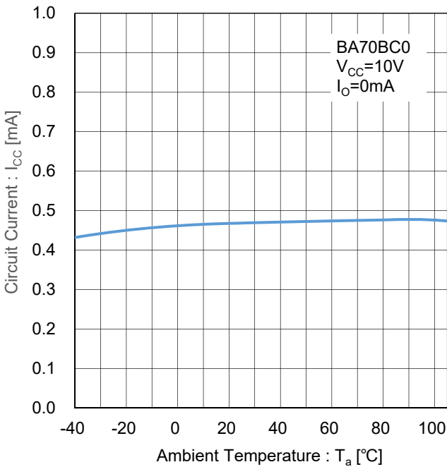
Figure 116. 回路電流 vs 温度 Test Circuit I
