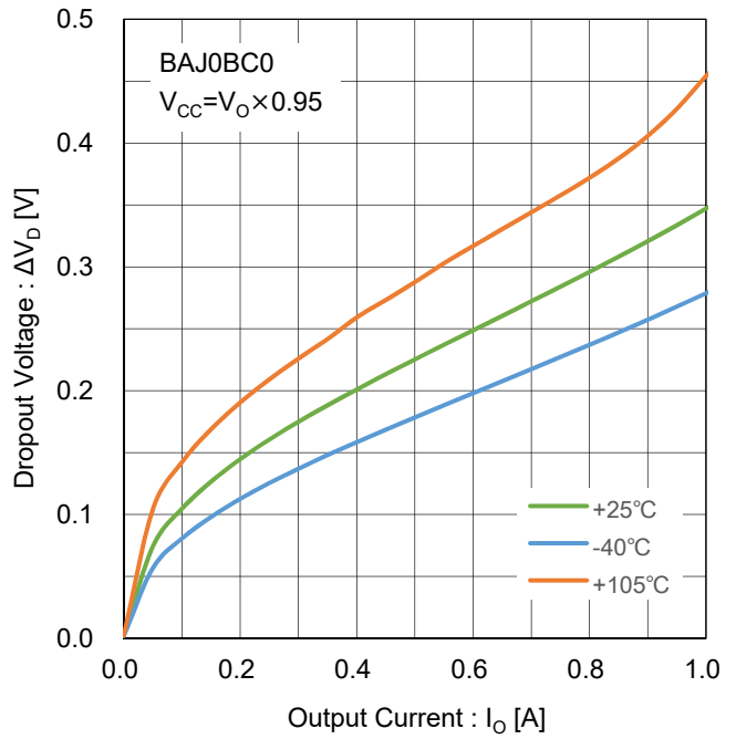
Figure 152. 最小入出力電圧差 vs 出力電流 Test Circuit B
