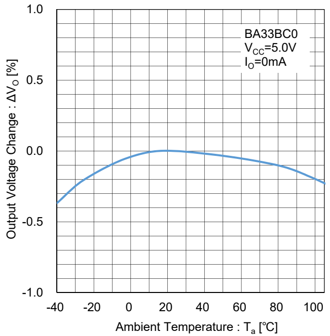
Figure 70. 出力電圧温度安定性 Test Circuit H
