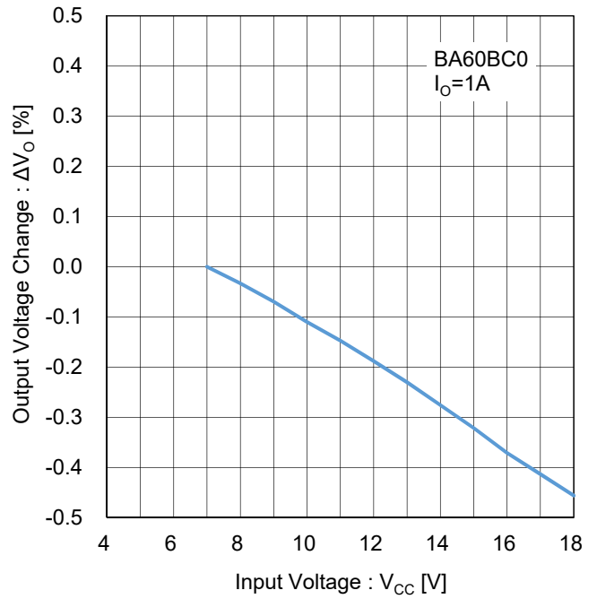
Figure 96. ラインレギュレーション ( I_O=1A ) Test Circuit D
