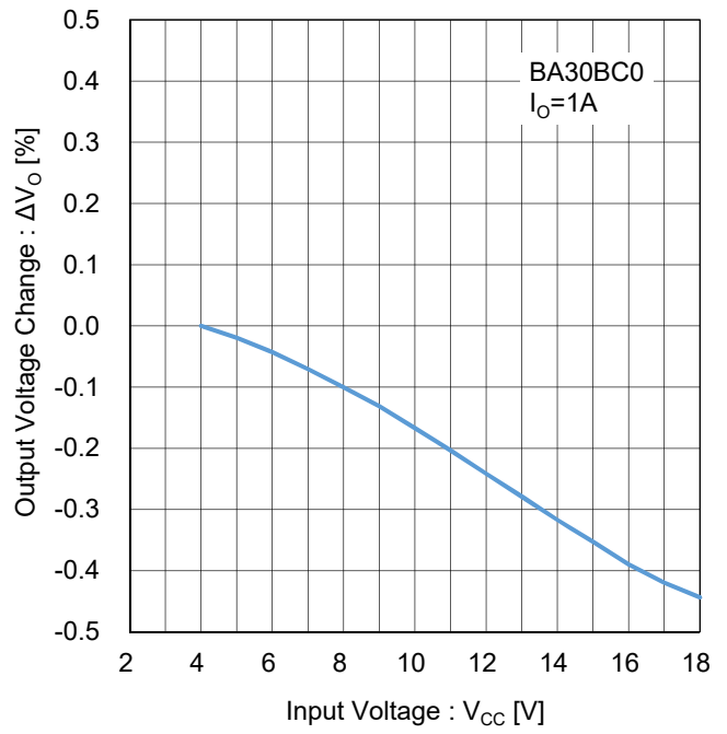
Figure 51. ラインレギュレーション ( I_o=1A ) Test Circuit D
