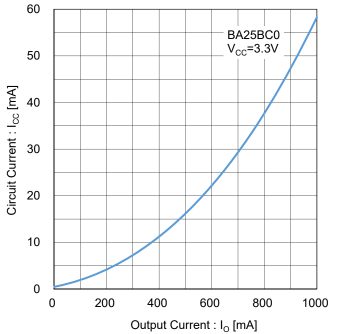
Figure 42. 回路電流 vs 出力電流 Test Circuit J
