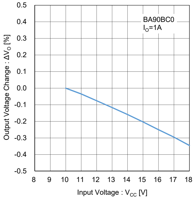
Figure 141. ラインレギュレーション ( I_o=1A ) Test Circuit D
