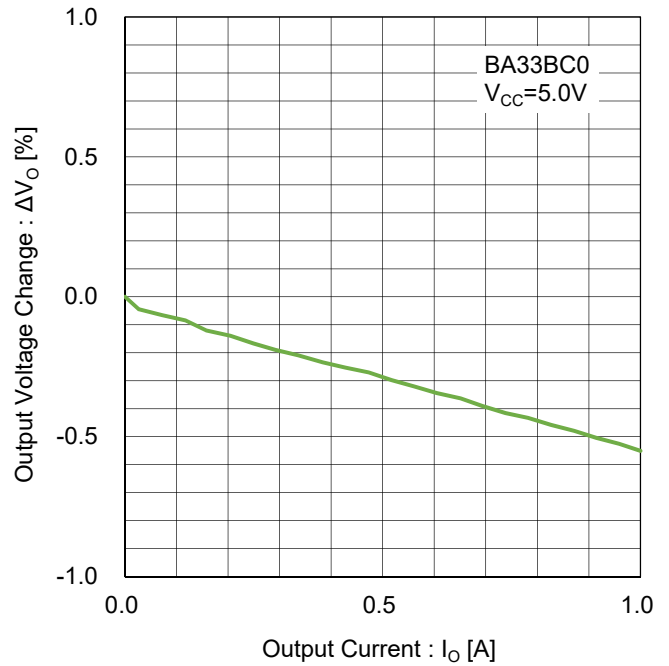
Figure 68. ロードレギュレーション Test Circuit F
