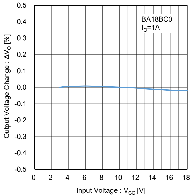
Figure 21. ラインレギュレーション ( I_o=1A ) Test Circuit D
