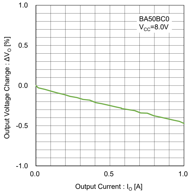
Figure 83. ロードレギュレーション Test Circuit F
