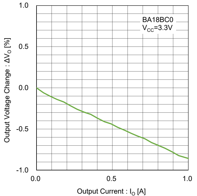
Figure 23. ロードレギュレーション Test Circuit F
