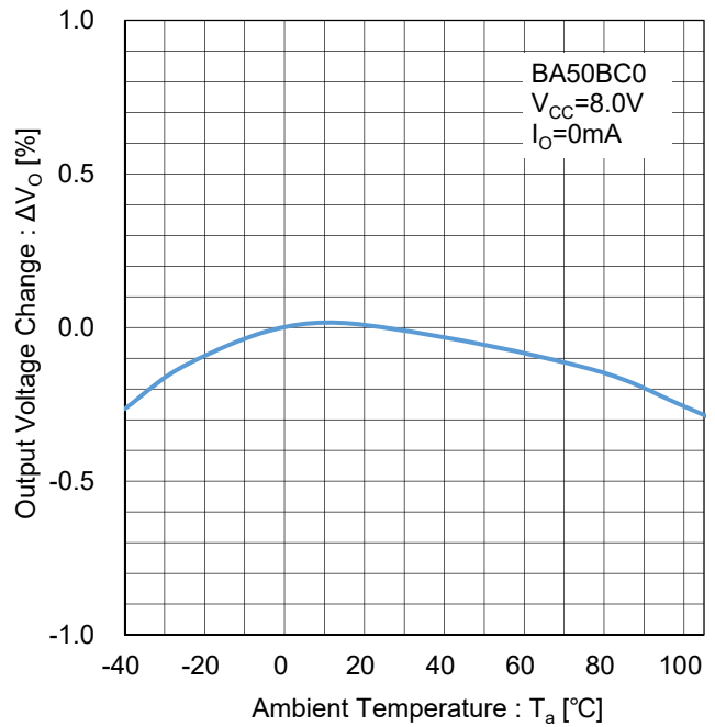
Figure 85. 出力電圧温度安定性 Test Circuit H
