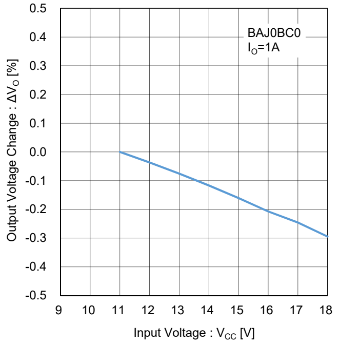
Figure 156. ラインレギュレーション ( I_o=1A ) Test Circuit D
