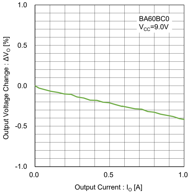
Figure 98. ロードレギュレーション Test Circuit F
