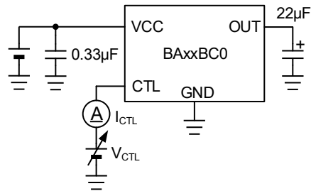
Test Circuit L. CTL ピン流入電流
