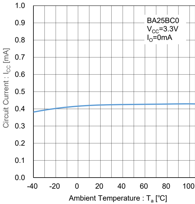
Figure 41. 回路電流 vs 温度 Test Circuit I
