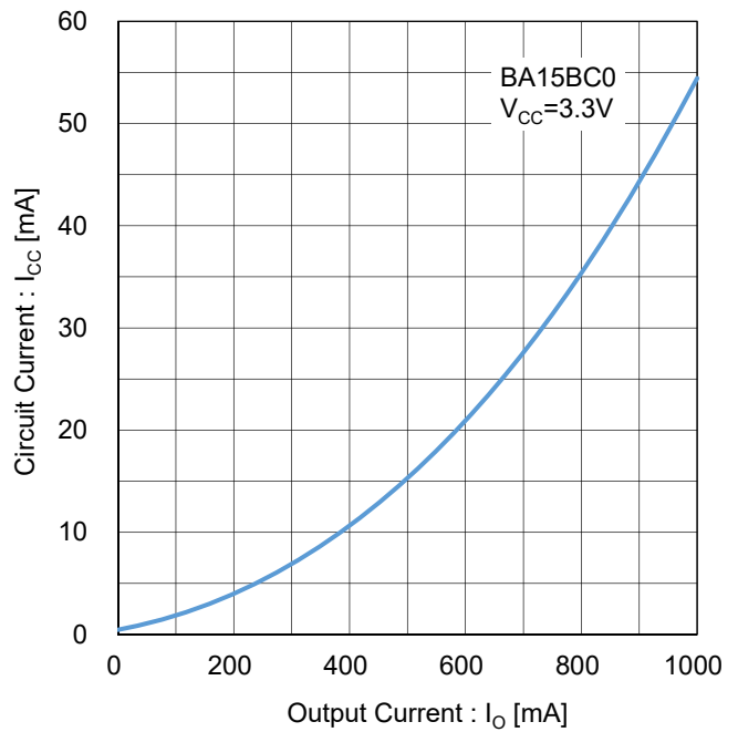
Figure 12. 回路電流 vs 出力電流 Test Circuit J
