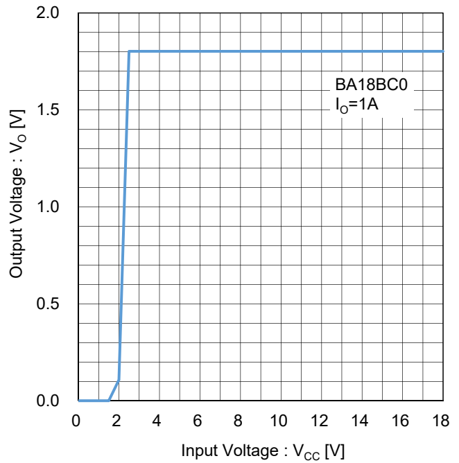
Figure 19. 出力電圧 vs 入力電圧 ( I_o=1A ) Test Circuit C
