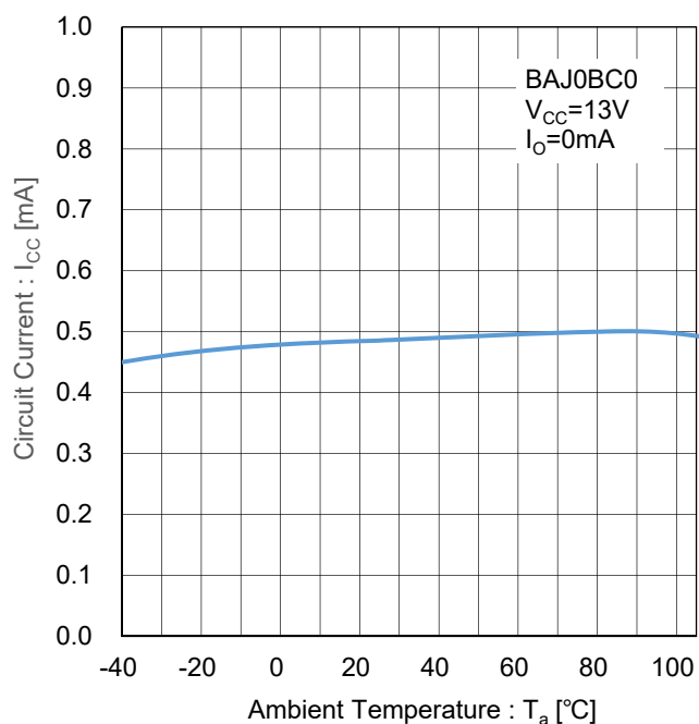
Figure 161. 回路電流 vs 温度 Test Circuit I
