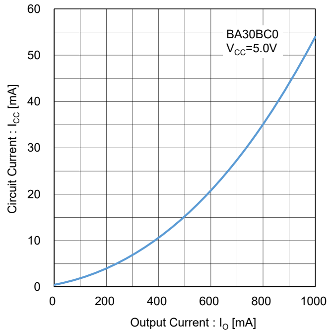
Figure 57. 回路電流 vs 出力電流 Test Circuit J
