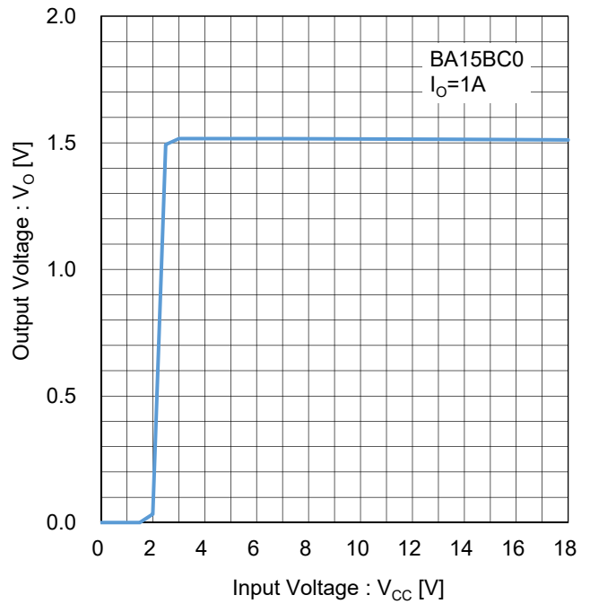
Figure 4. 出力電圧 vs 入力電圧 ( I_o=1A ) Test Circuit C
