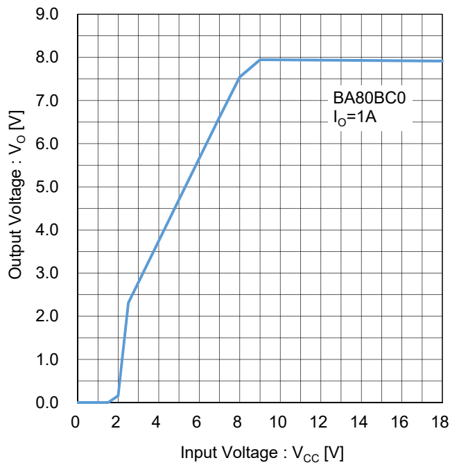
Figure 124. 出力電圧 vs 入力電圧 ( I_O=1A ) Test Circuit C
