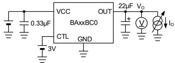
Test Circuit F. ロードレギュレーション
