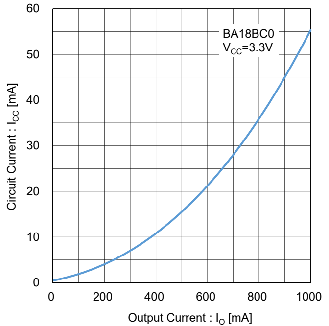
Figure 27. 回路電流 vs 出力電流 Test Circuit J
