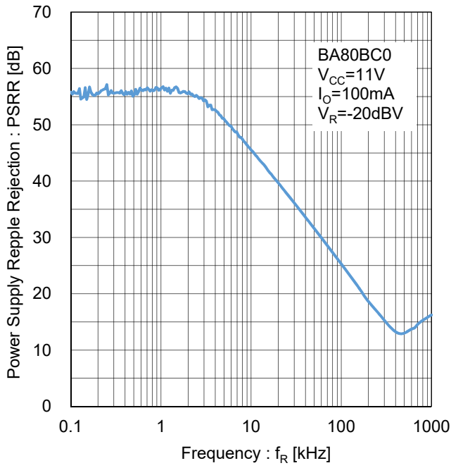
Figure 129. リップルリジェクション Test Circuit G
