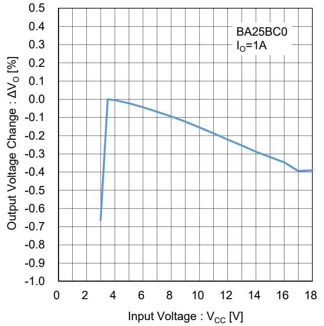
Figure 36. ラインレギュレーション ( I_o=1A ) Test Circuit D
