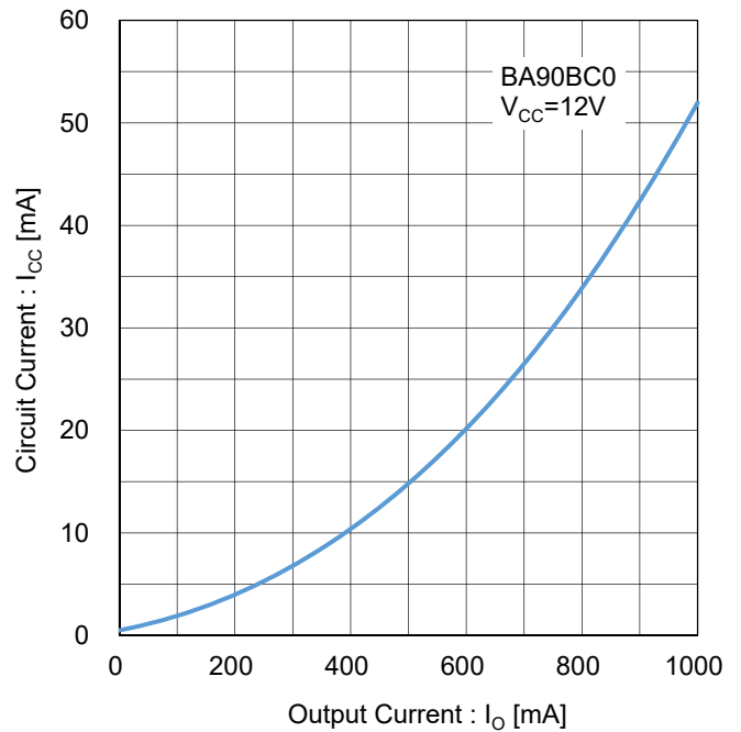
Figure 147. 回路電流 vs 出力電流 Test Circuit J
