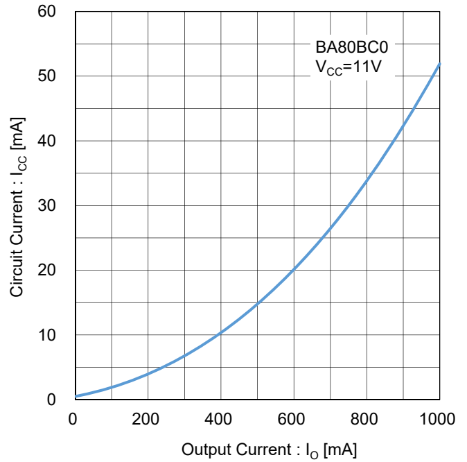
Figure 132. 回路電流 vs 出力電流 Test Circuit J
