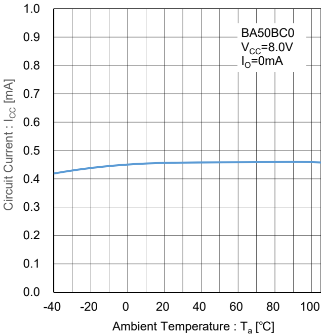
Figure 86. 回路電流 vs 温度 Test Circuit I
