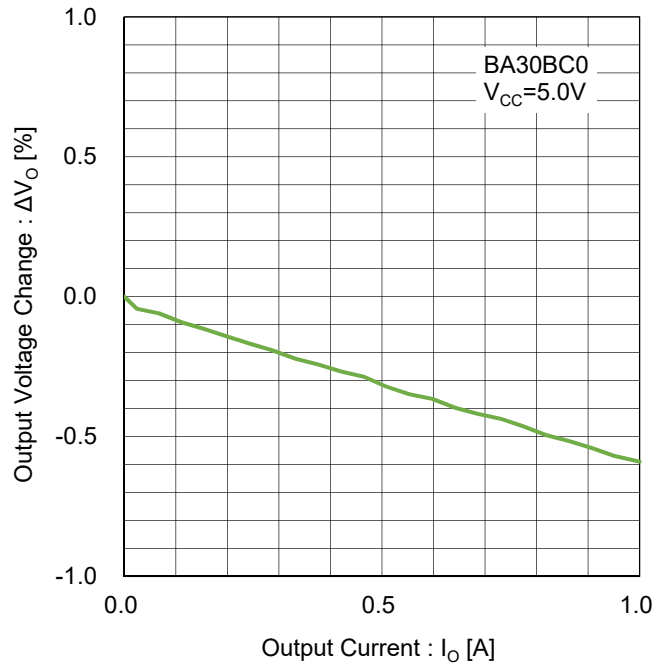
Figure 53. ロードレギュレーション Test Circuit F
