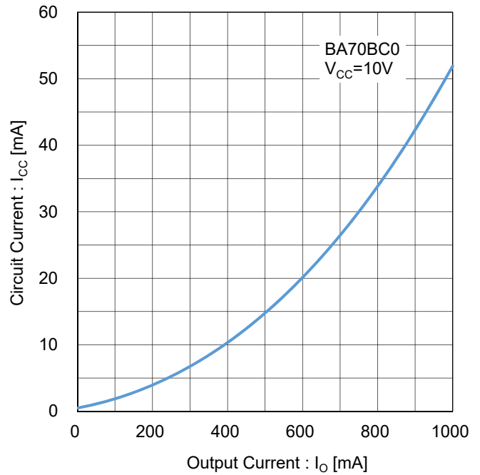
Figure 117. 回路電流 vs 出力電流 Test Circuit J
