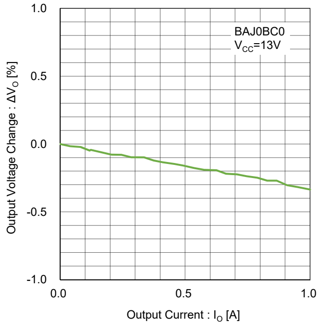
Figure 158. ロードレギュレーション Test Circuit F
