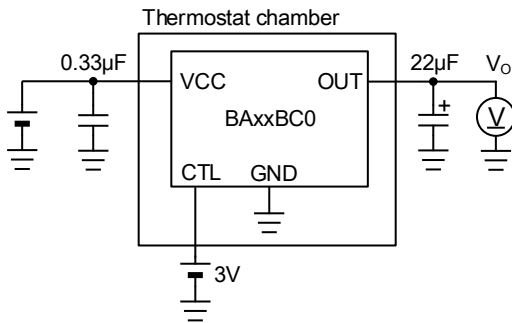
Test Circuit M. 過熱保護
