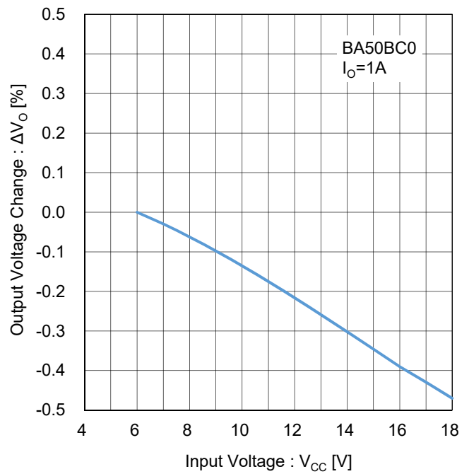
Figure 81. ラインレギュレーション ( I_o=1A ) Test Circuit D
