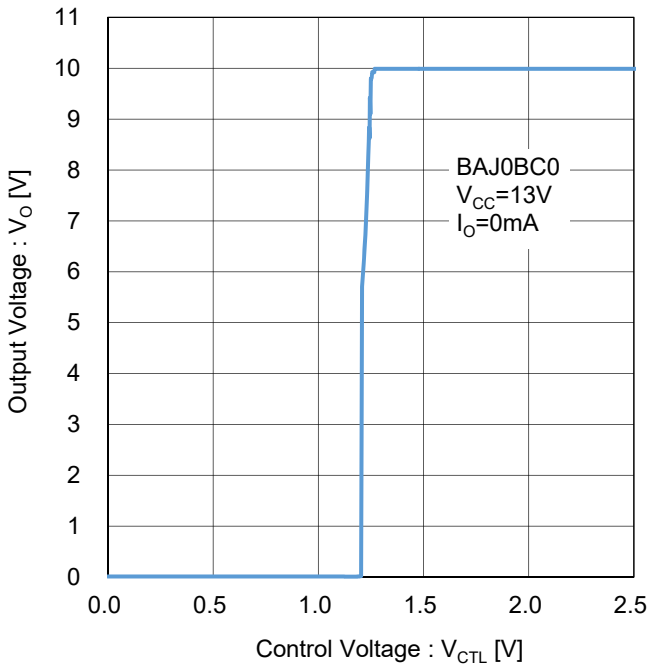
Figure 163. 出力電圧 vs CTL ピン電圧 Test Circuit K
