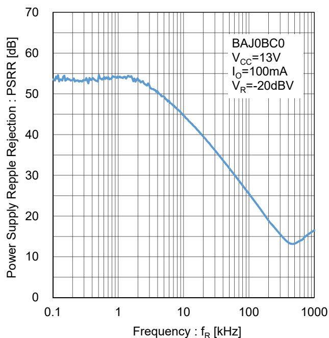
Figure 159. リップルリジェクション Test Circuit G
