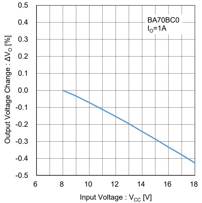
Figure 111. ラインレギュレーション ( I_o=1A ) Test Circuit D
