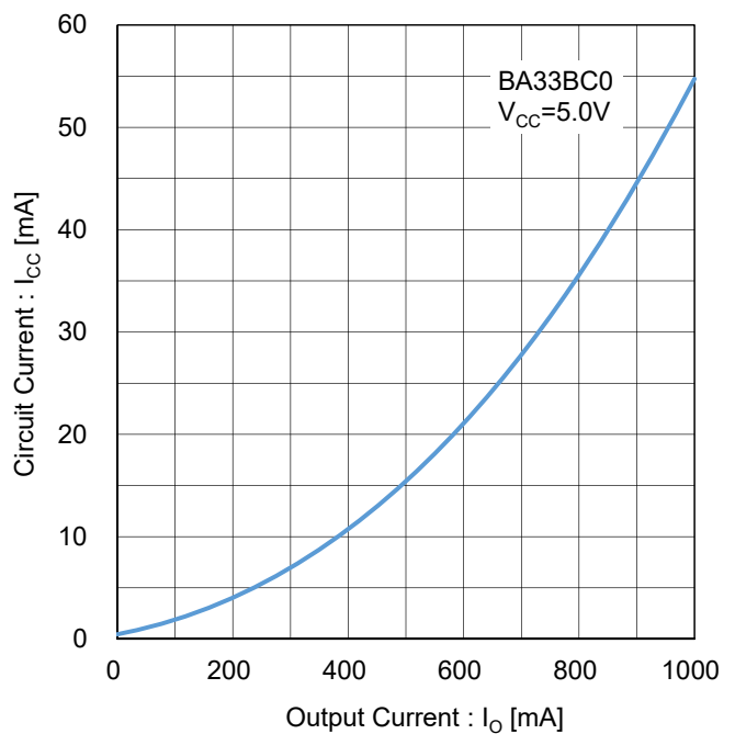
Figure 72. 回路電流 vs 出力電流 Test Circuit J
