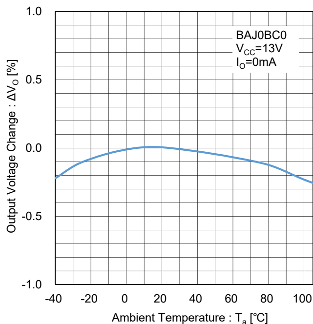
Figure 160. 出力電圧温度安定性 Test Circuit H
