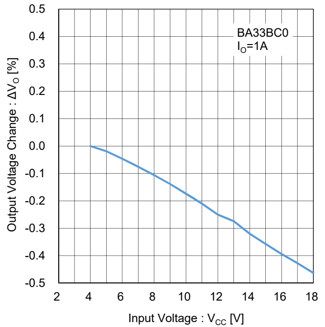
Figure 66. ラインレギュレーション ( I_O=1A ) Test Circuit D
