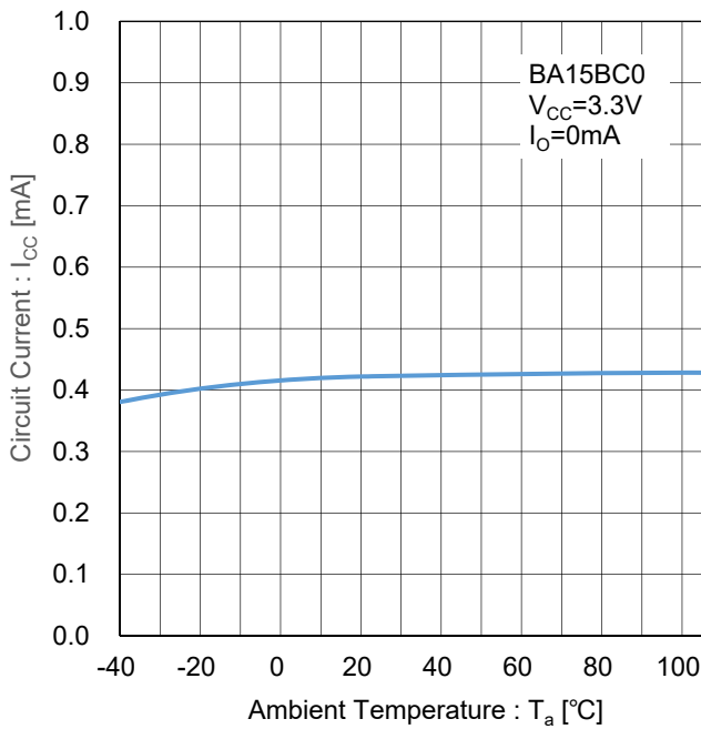
Figure 11. 回路電流 vs 温度 Test Circuit I
