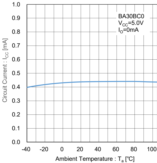
Figure 56. 回路電流 vs 温度 Test Circuit I
