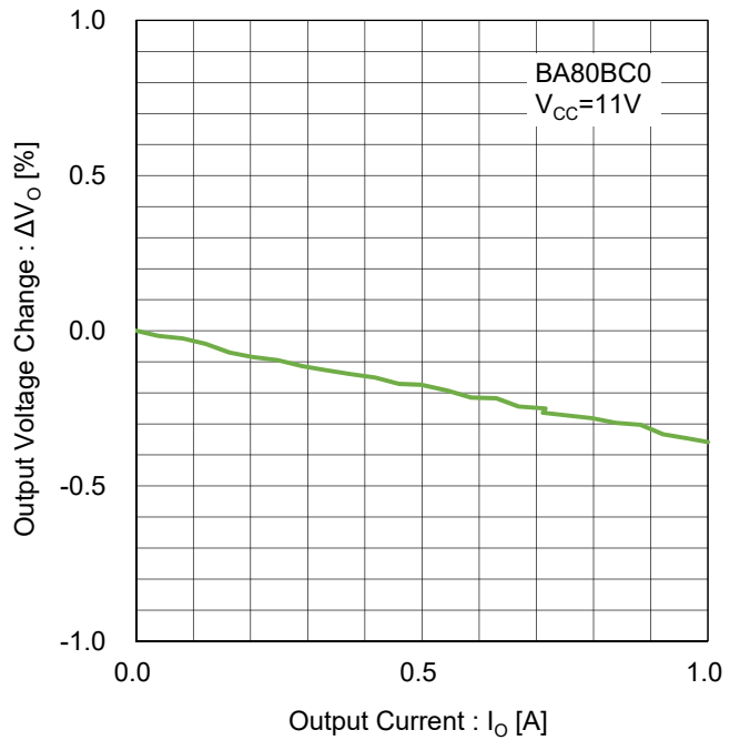
Figure 128. ロードレギュレーション Test Circuit F
