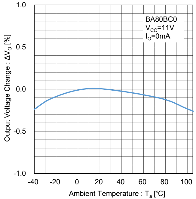
Figure 130. 出力電圧温度安定性 Test Circuit H
