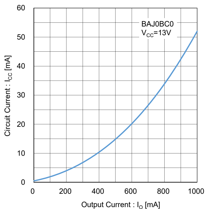
Figure 162. 回路電流 vs 出力電流 Test Circuit J
