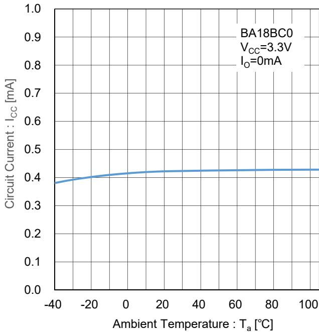
Figure 26. 回路電流 vs 温度 Test Circuit I
