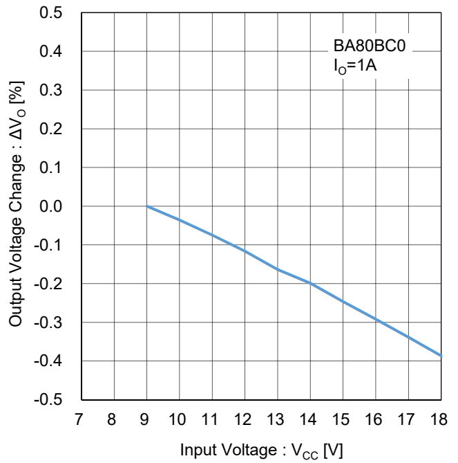
Figure 126. ラインレギュレーション ( I_o=1A ) Test Circuit D
