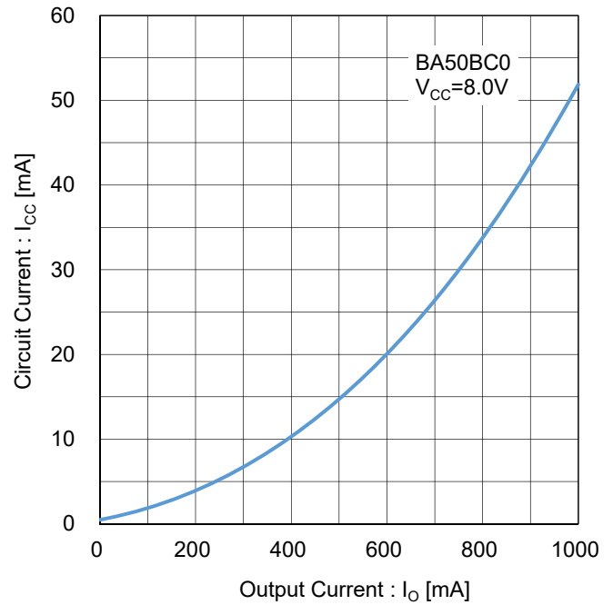
Figure 87. 回路電流 vs 出力電流 Test Circuit J
