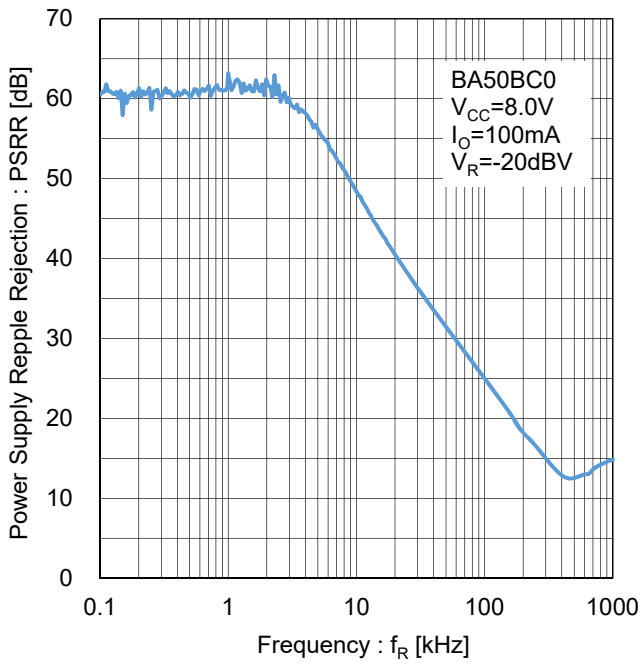
Figure 84. リップルリジエクション Test Circuit G
