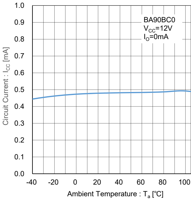
Figure 146. 回路電流 vs 温度 Test Circuit I
