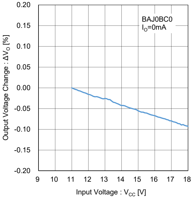
Figure 155. ラインレギュレーション ( I_o=0mA ) Test Circuit D
