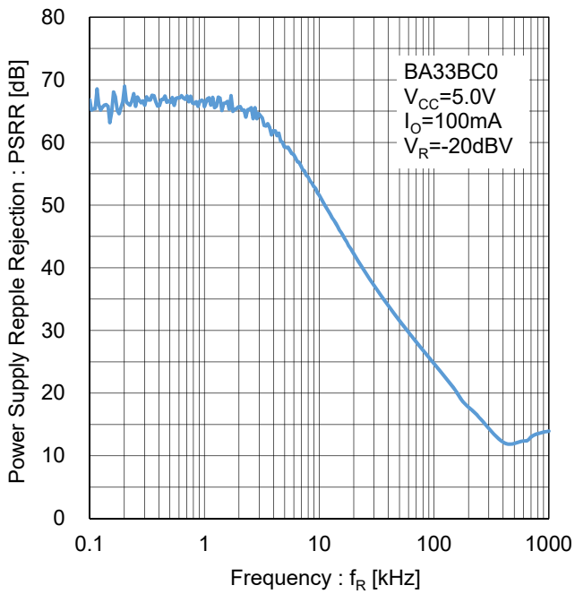
Figure 69. リップルリジェクション Test Circuit G
