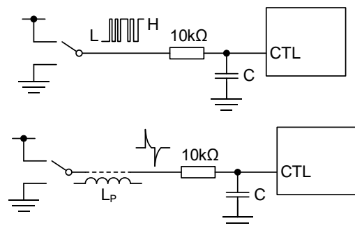
Figure 6-3. CTL ピンの RC フィルタ回路
