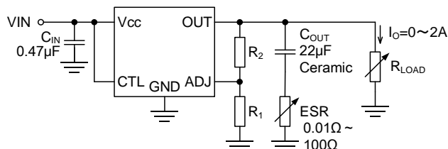
Figure 7-2. ESR 安定動作領域評価回路
