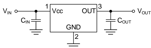
Figure 1-9. 代表的なアプリケーション回路
