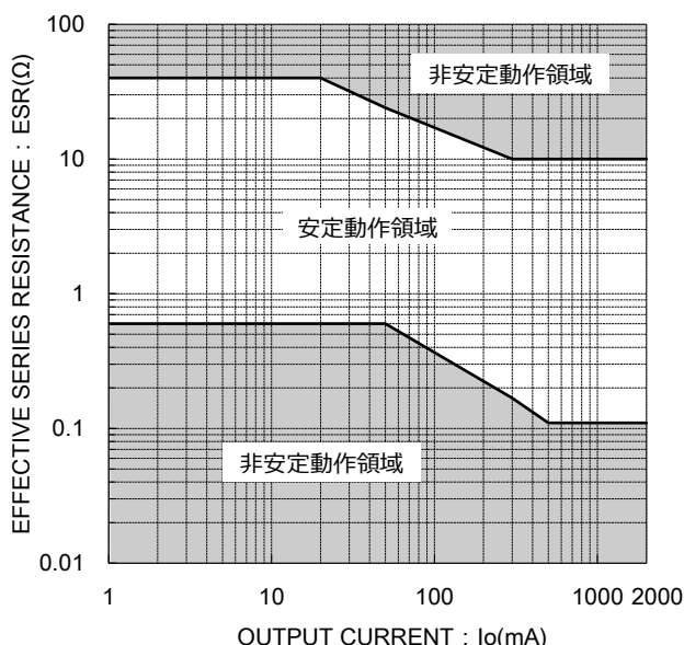
Figure 7-1. ESR 安定動作領域
