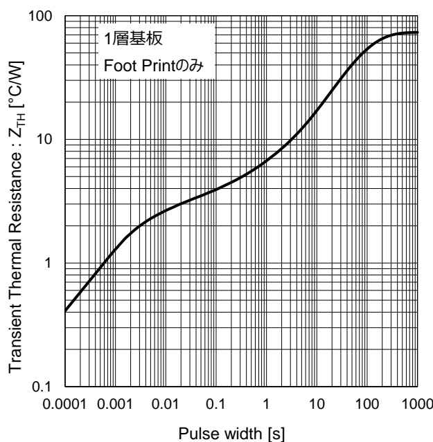
Figure 15-2. HRP5 パッケージの過渡熱抵抗
