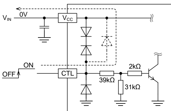
Figure 6-1. CTL を先に立ち上げる場合の制限抵抗
