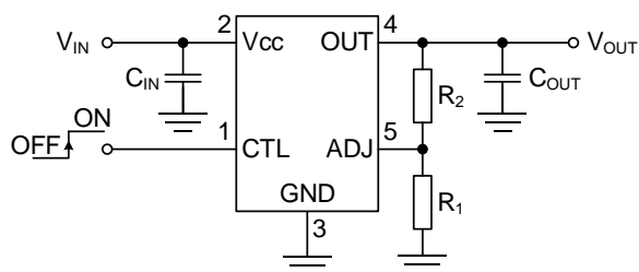
Figure 1-1. 出力 ON/OFF 機能を使用するとき
