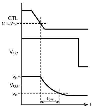
Figure 14-2. CTLを緩やかにオフした場合
