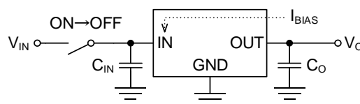
Figure 12-2. 入力をオープンにした場合
