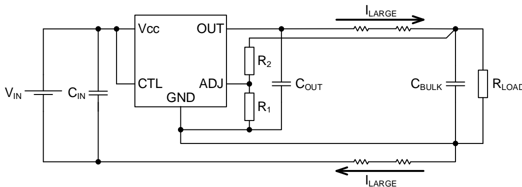
Figure 3-1. ケルビン接続
