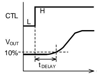
Figure 6-2. 起動遅延時間の定義
