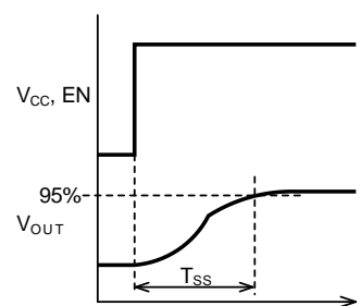
Figure 14-11. 途中で過電流保護回路により電流制限を受けた状態で起動した場合
