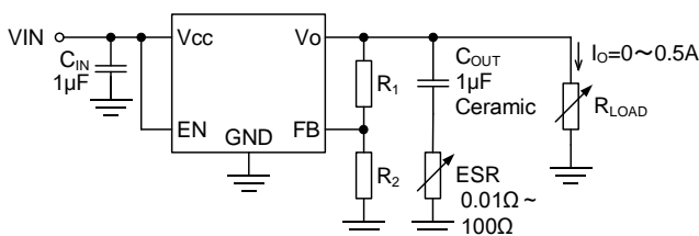
Figure 7-2. ESR 安定動作領域評価回路
