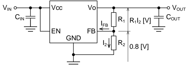
Figure 2-1. 出力電圧設定
