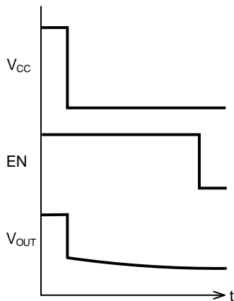
Figure 15-3. V_{CC} を急峻にオフした場合
