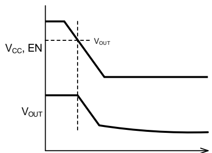
Figure 15-7. V_{CC} , EN を緩やかにオフした場合
