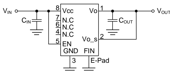
Figure 1-4. 出力 ON/OFF 機能を使用しないとき
