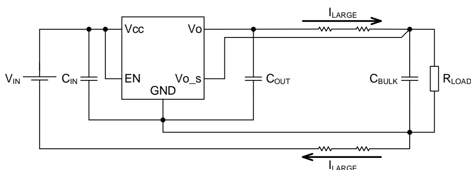
Figure 3-2. ケルビン接続 (固定出力型)
