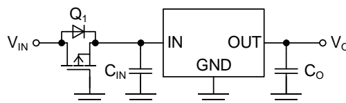
Figure 12-8. 逆接続対策 4
