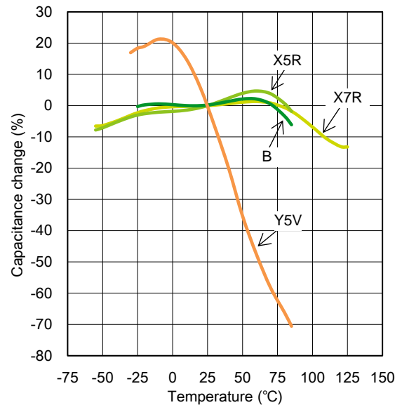
Figure 7-3. 主な高誘電率系積層セラミックコンデンサの温度特性
