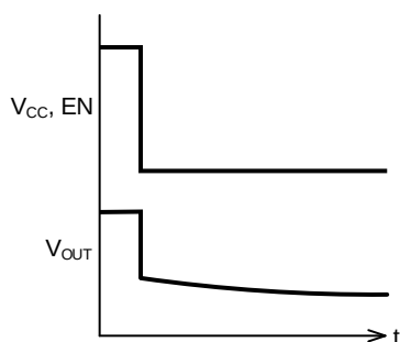
Figure 15-6. V_{CC} , EN を急峻にオフした場合
