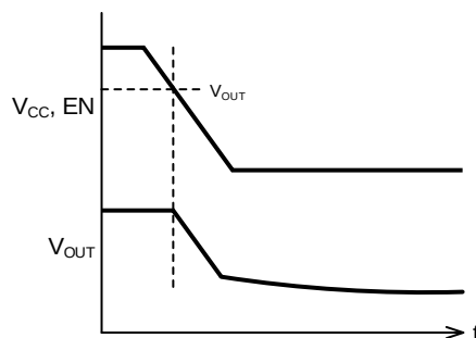
Figure 15-7. V_{CC} , EN を緩やかにオフした場合
