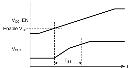
Figure 14-9. V_{CC} , EN をソフトスタート時間 よりも遅くオンした場合
