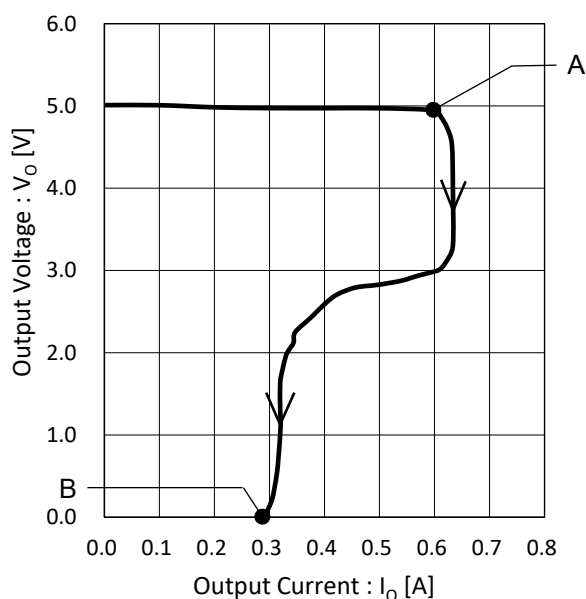
Figure 17-1. 過電流保護特性
