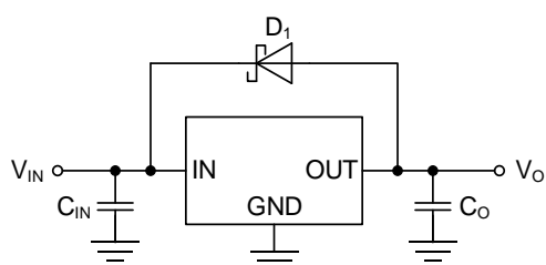
Figure 12-1. 逆電流バイパスダイオード
