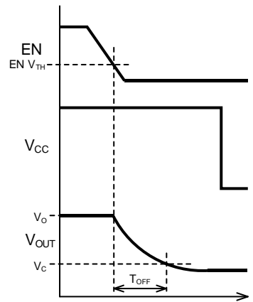
Figure 15-2. EN を緩やかにオフした場合
