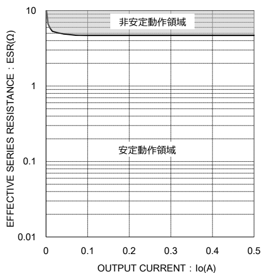
Figure 7-1. ESR 安定動作領域
