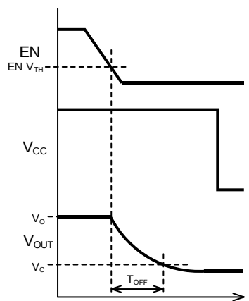
Figure 15-2. EN を緩やかにオフした場合
