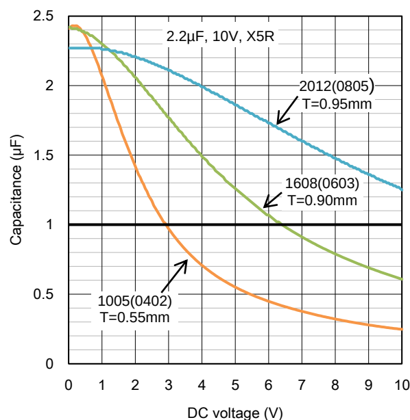
Figure 7-4. 高誘電率系積層セラミックコンデンサの DC バイアス特性、サイズによる比較
