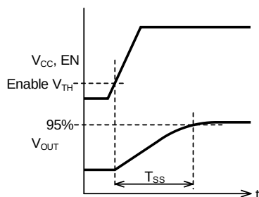
Figure 14-8. V_{CC} , EN をソフトスタート時間 よりも速くオンした場合
