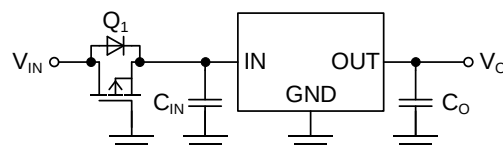
Figure 12-8. 逆接続対策 4
