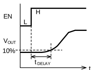
Figure 6-1. 起動遅延時間の定義
