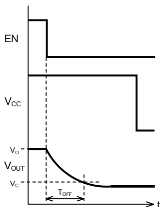
Figure 15-1. EN を急峻にオフした場合
