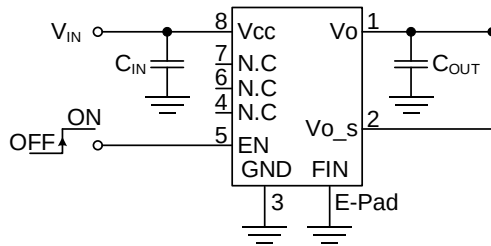
Figure 1-3. 出力 ON/OFF 機能を使用するとき
