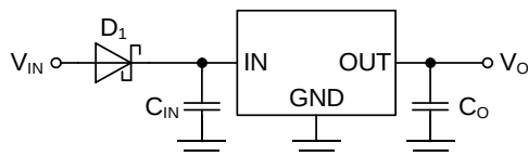
Figure 12-5. 逆接続対策 1
