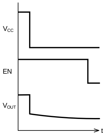
Figure 15-3. V_{CC} を急峻にオフした場合
