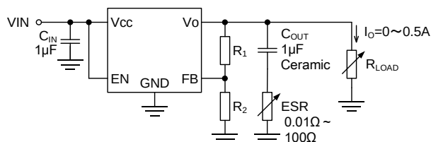
Figure 7-2. ESR 安定動作領域評価回路
