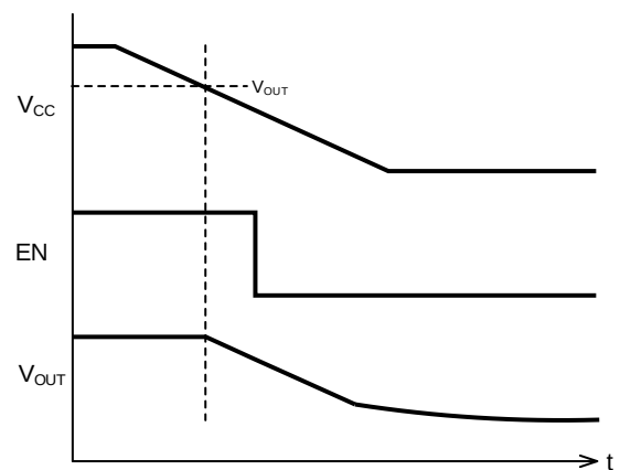
Figure 15-5. V_{CC} を緩やかにオフし、さらに V_{CC} 降下中に EN をオフした場合
