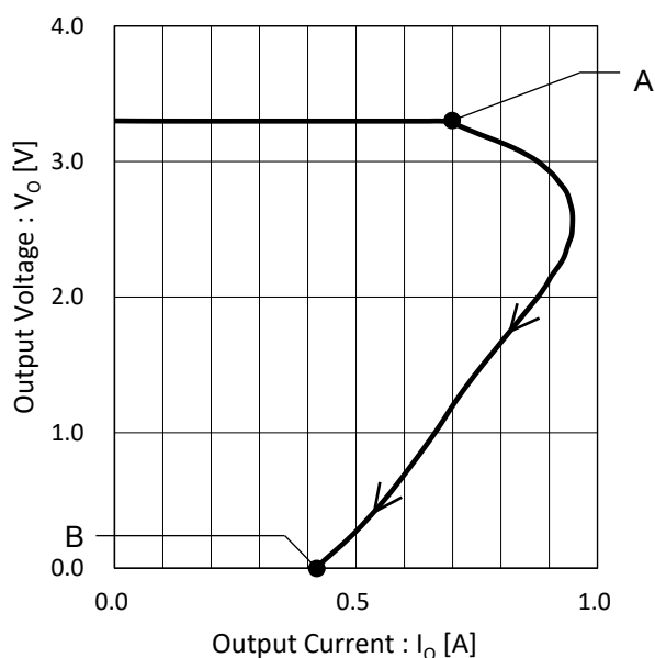
Figure 17-1. 過電流保護特性
