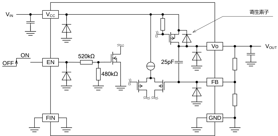
Figure 19-1. 可変出力型等価回路
