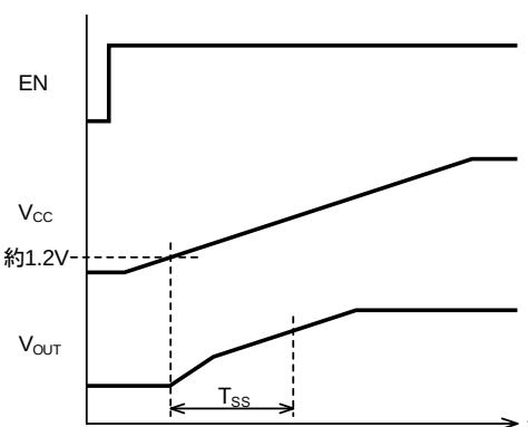
Figure 14-6. V CC をソフトスタート時間 よりも遅くオンした場合
