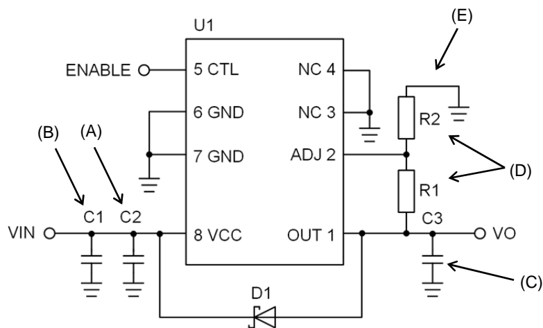
Figure 8. 回路図 (可変出力タイプ)
