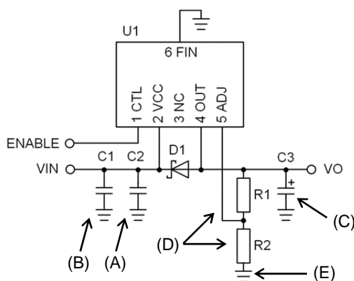
Figure 4. 回路図 (可変出力タイプ)
