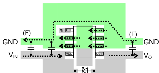
Figure 13. 大電流グラウンド配線
