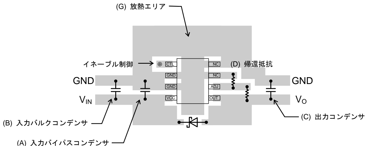
Figure 5. PCB レイアウト (HTSOP-J8 パッケージ)
