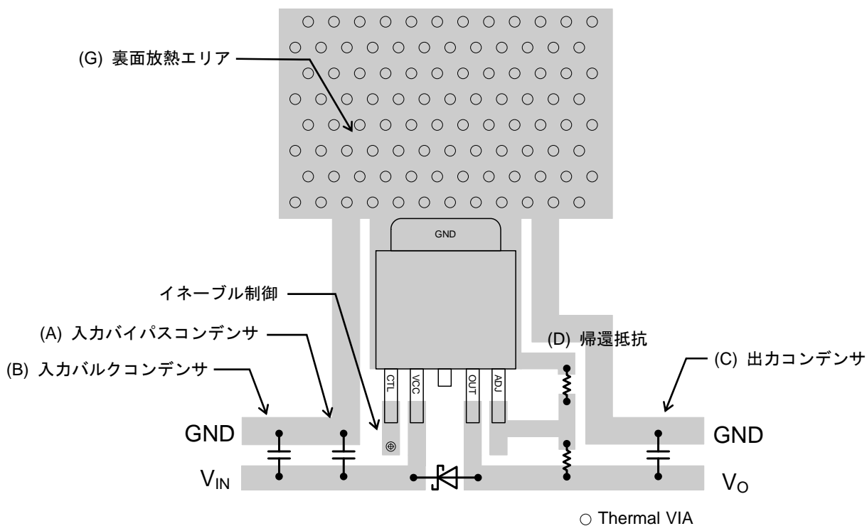
Figure 1. PCB レイアウト (TO252-5 パッケージ)
