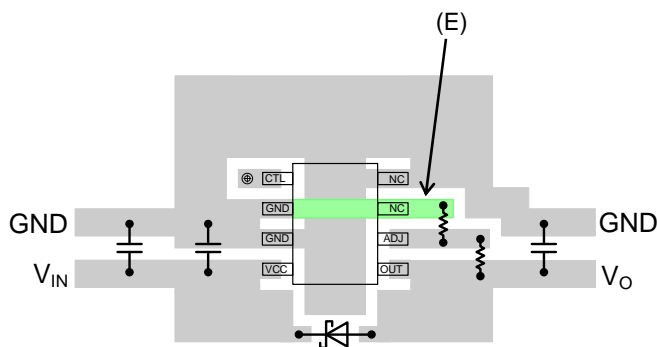
Figure 6. 小信号グラウンド配線
