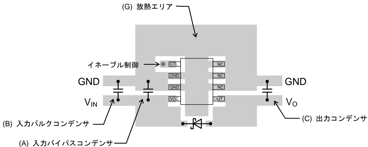
Figure 12. PCB レイアウト (HTSOP-J8 パッケージ)
