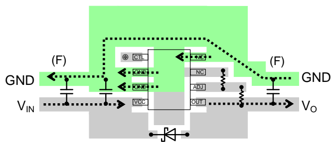
Figure 7. 大電流グラウンド配線
