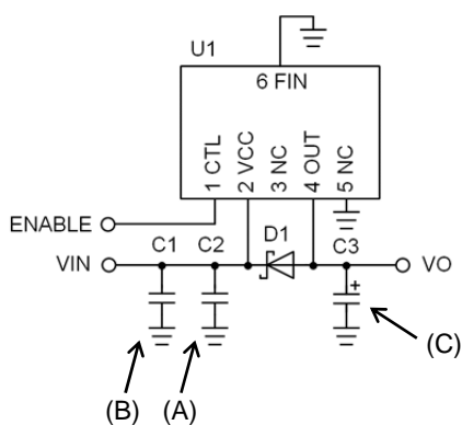
Figure 11. 回路図 (固定出力タイプ)
