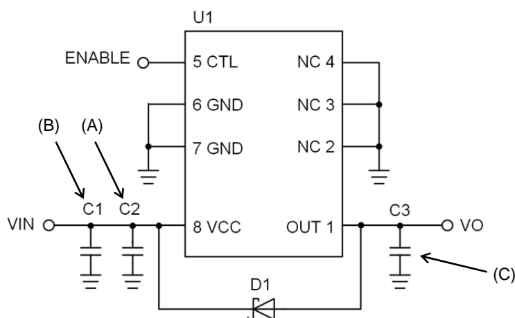
Figure 14. 回路図 (固定出力タイプ)
