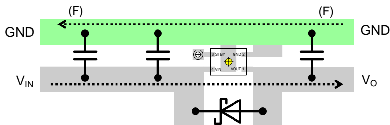
Figure 5. 大電流グラウンド配線
