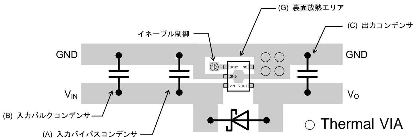
Figure 1. PCB レイアウト (HVSOF5 パッケージ)
