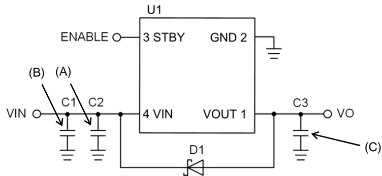
Figure 6. 回路図
