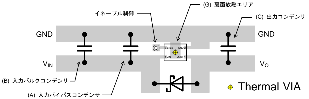
Figure 4. PCB レイアウト (SSON004X1216 パッケージ)
