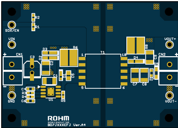
Figure 5. Top シルクスクリーン, レイアウト (Top View)
