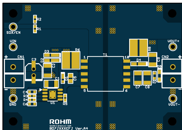
Figure 13. Top ランドパターン (Top View)
