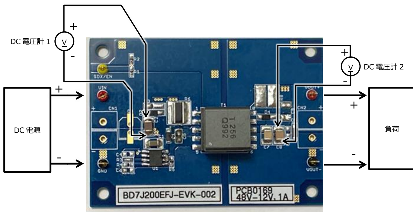
Figure 3. 接続図
