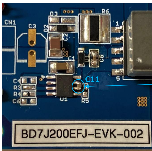
Figure 14. C11 取り付け位置
