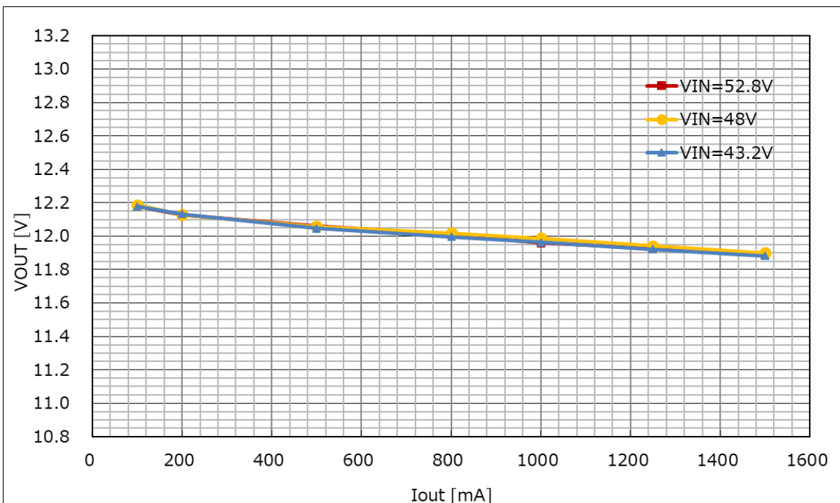
Figure 12. ロードレギュレーション
