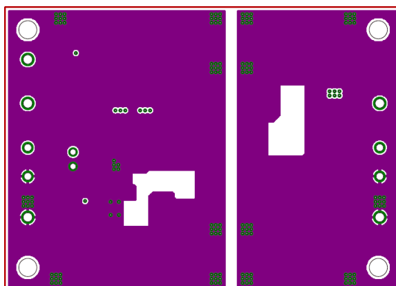
Figure 9. Middle Layer2 レイアウト (Top View)
