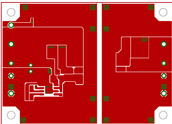
Figure 7. Top Layer レイアウト (Top View)
