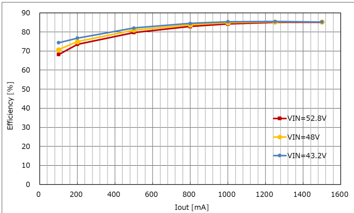
Figure 11. 電力変換効率 vs 負荷電流
