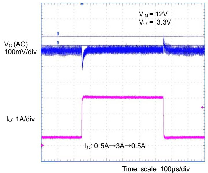
Figure 12. 負荷過渡特性
