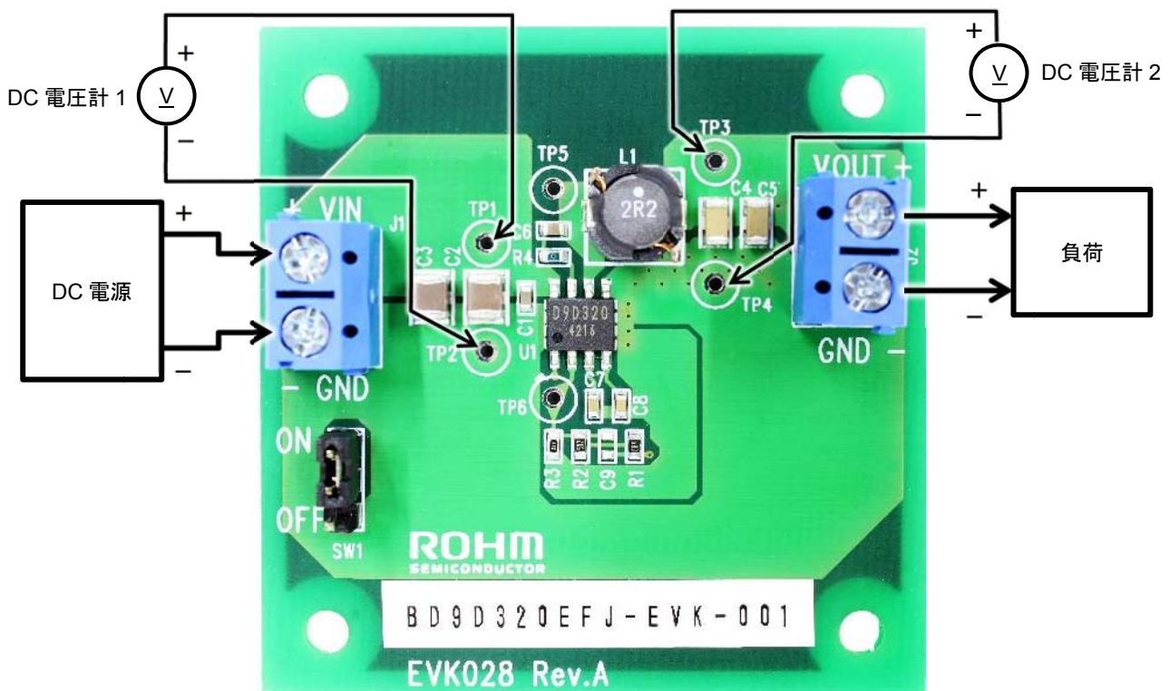
Figure 1. 接続図
