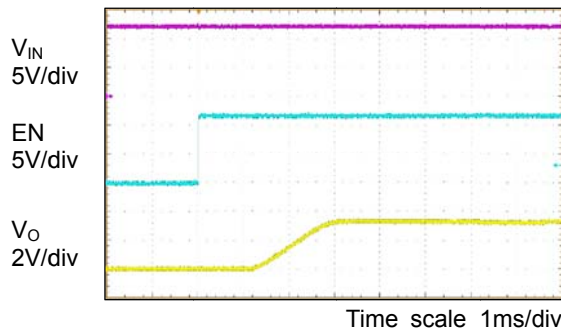
Figure 17. スタートアップ EN による V_{IN} = 12V, V_O = 3.3V, I_O = 0A
