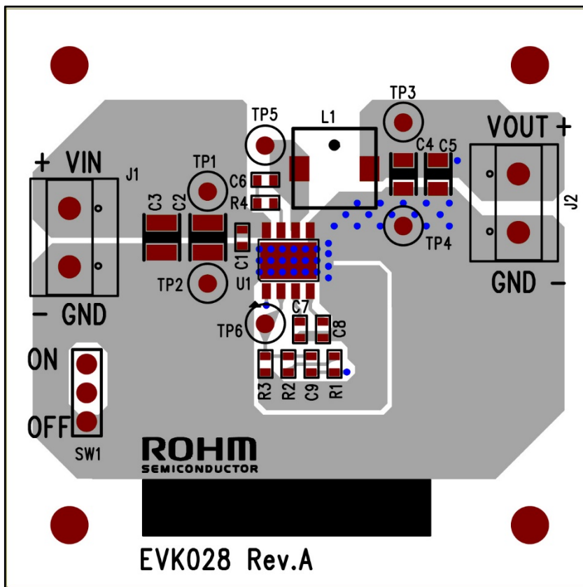
Figure 4. Top シルksスクリーンとレイアウト (Top view)
