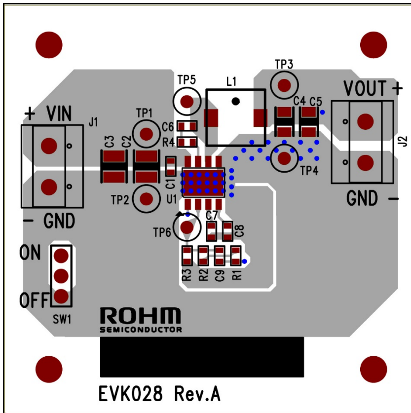
Figure 4. Top シルクスクリーンとレイアウト (Top view)
