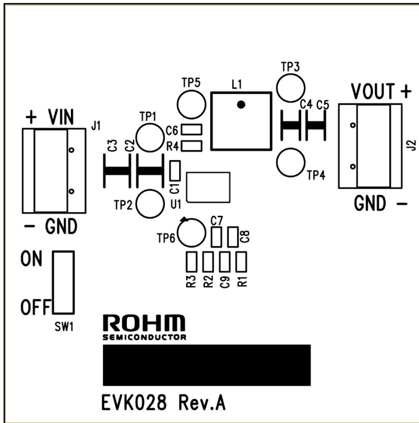
Figure 3. Top シルクスクリーン (Top view)
