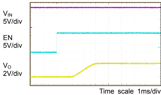
Figure 17. スタートアップ ENによる V_{IN} = 12V, V_O = 3.3V, I_o = 0A
