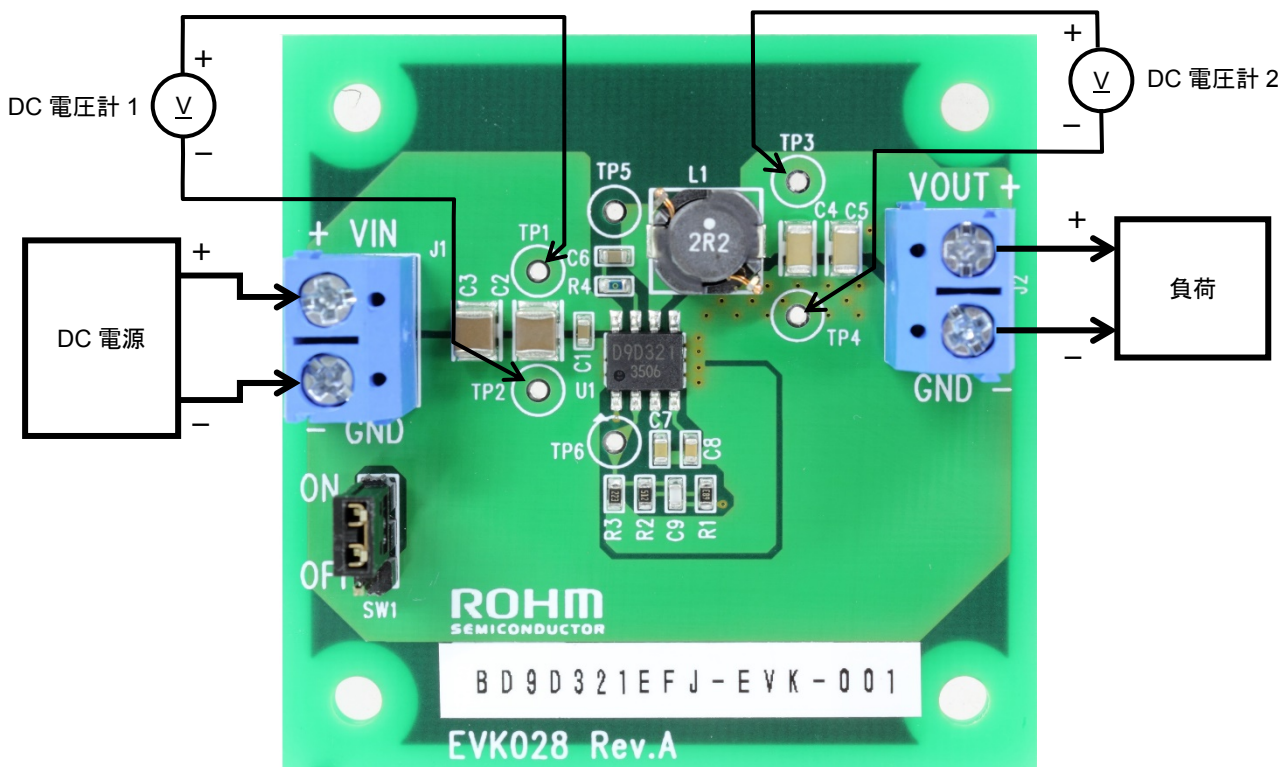
Figure 1. 接続図
