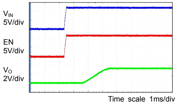
Figure 15. スタートアップ EN = V_{IN} V_{IN} = 12V, V_O = 3.3V, I_o = 0A
