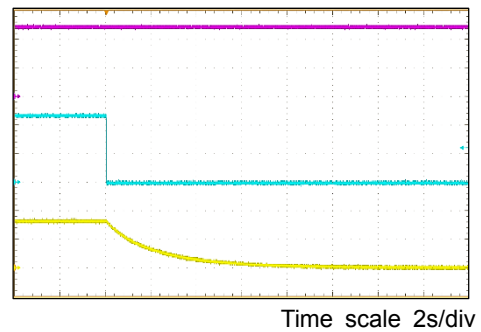
Figure 18. パワーダウン ENによる V_{IN} = 12V, V_O = 3.3V, I_o = 0A
