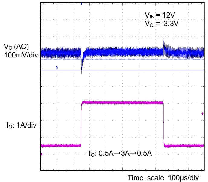
Figure 12. 負荷過渡特性
