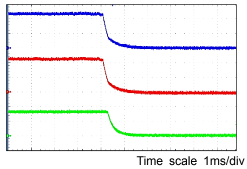
Figure 16. パワーダウン EN = V_{IN} V_{IN} = 12V, V_O = 3.3V, I_o = 0A
