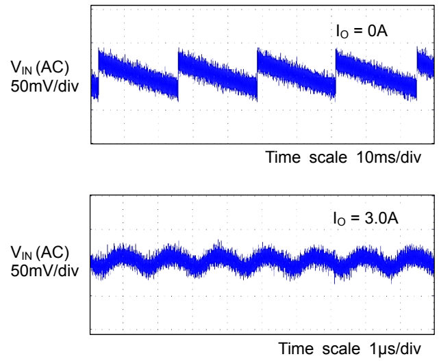
Figure 14. 出力電圧リップル波形 V_{IN} = 12V, V_O = 3.3V
