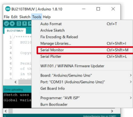
Figure 5. Tools 設定
