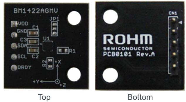
Figure 7. 基板の写真
