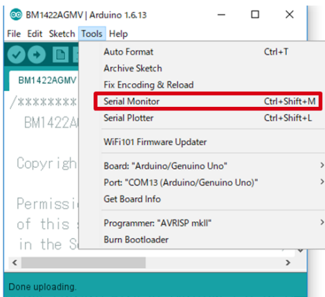
Figure 5. Tools 設定
