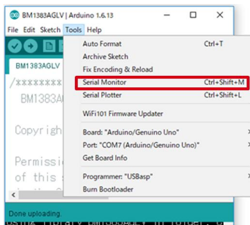
Figure 5. Tools 設定
