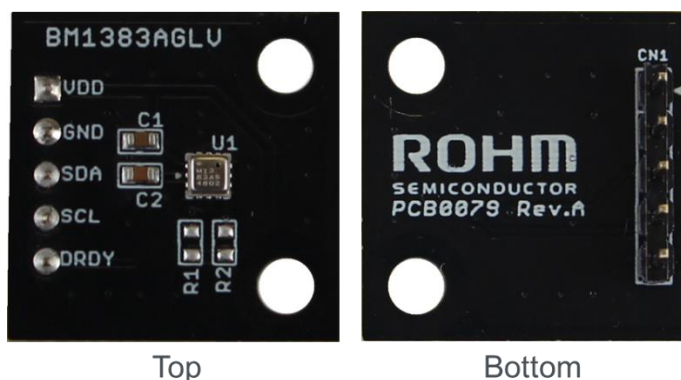
Figure 7. 基板の写真
