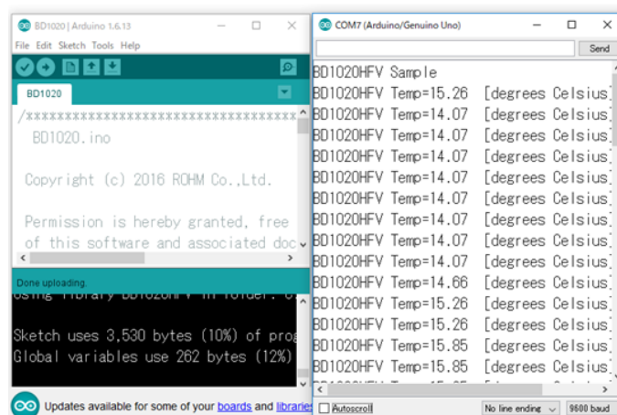
図 10 BD1020HFV (アナログセンサ)の実行画面
