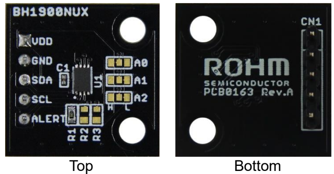
Figure 7. 基板の写真
