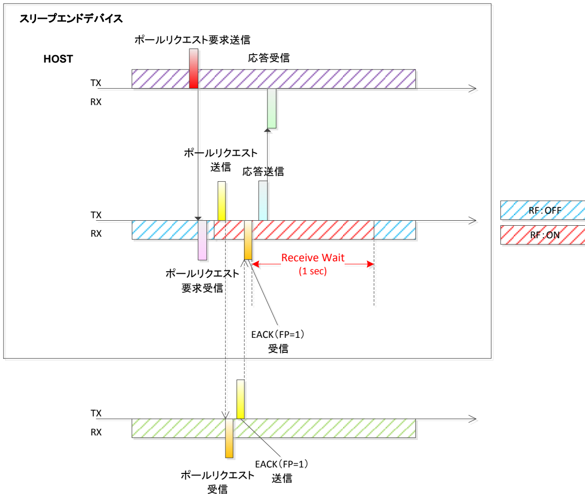
図 14 Poll Request 送信 ~ キューイングデータ受信タイムアウト
