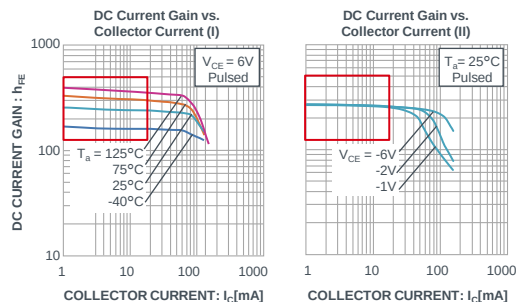
2SC4081U3 (NPN)
