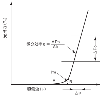
■Fig.2 光出力-順電流特性
