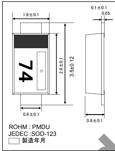
●外形寸法図 (Unit : mm)
