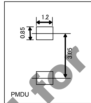
●推奨ランドパターン (Unit : mm)
